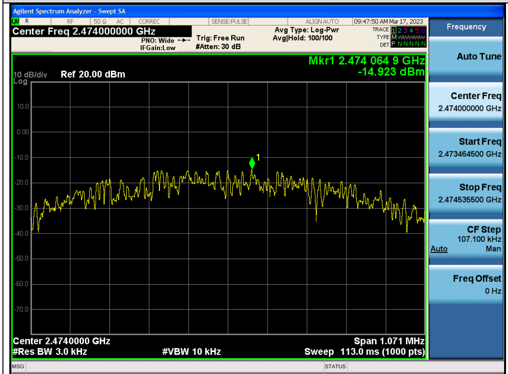
Test_Graph_GFSK_ANT1_2474_PSD
