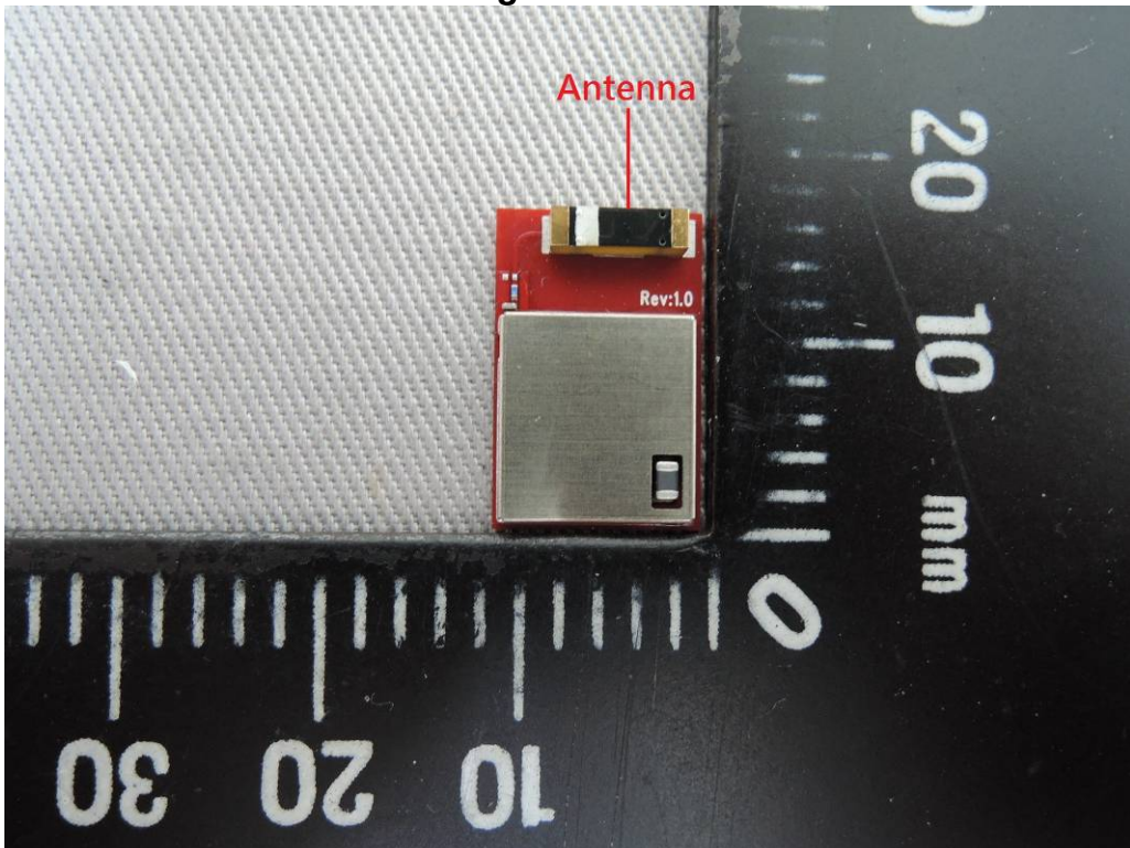
BT/Zigbee Antenna
