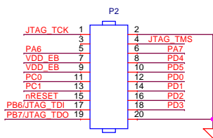
EM connector 2
