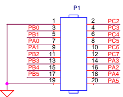
EM connector 1
