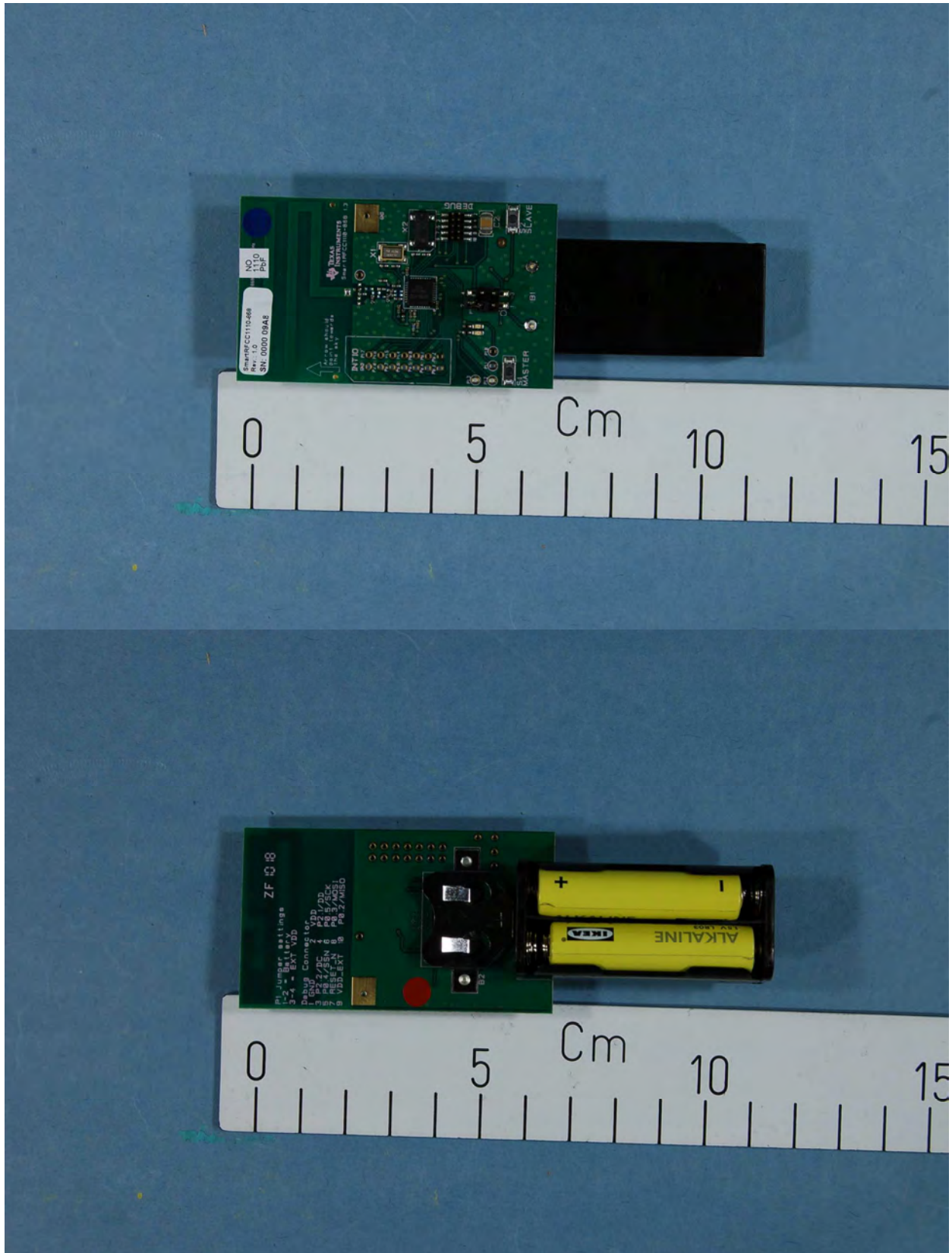
SmartRFCC1110EM
