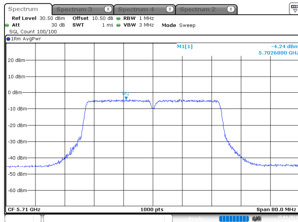
n40_5710MHz_Chain 2
