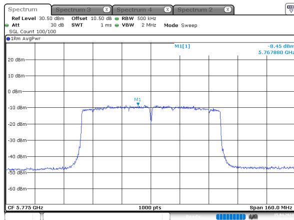
ac80_5775MHz_Chain 2
