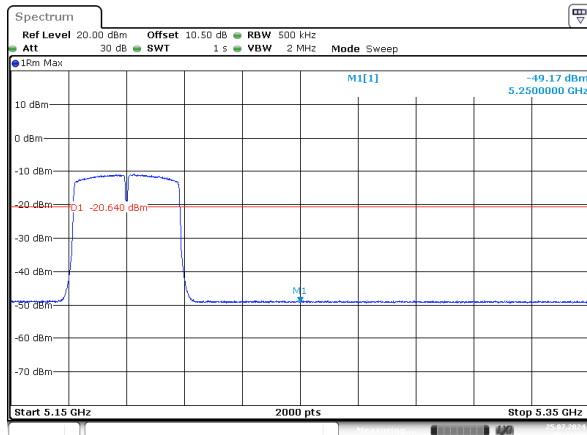
n40_5190MHz_Chain 0
