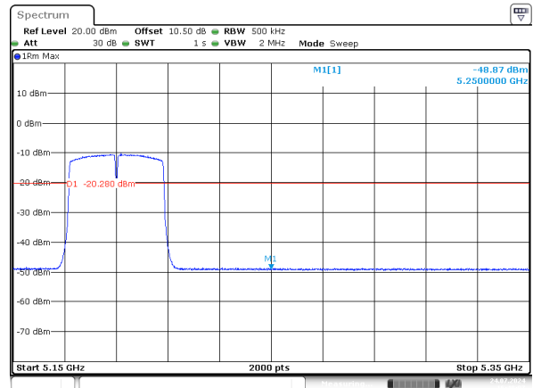
n40_5190MHz_Chain 1
