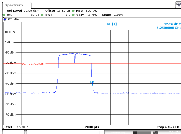
n40_5230MHz_Chain 0
