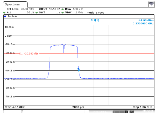
n40_5230MHz_Chain 1
