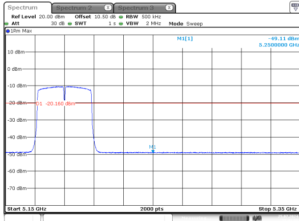
n40_5190MHz_Chain 2
