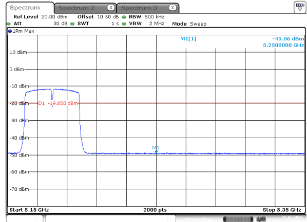
n40_5190MHz_Chain 3
