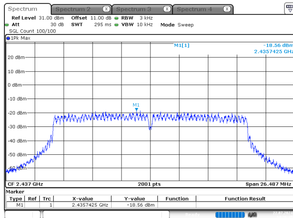
n20_2437MHz_Chain 2
