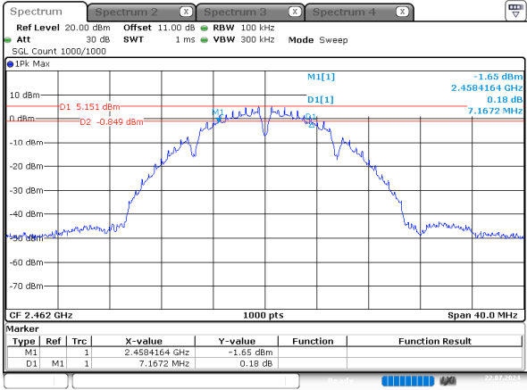
b_2462MHz_Chain 0
