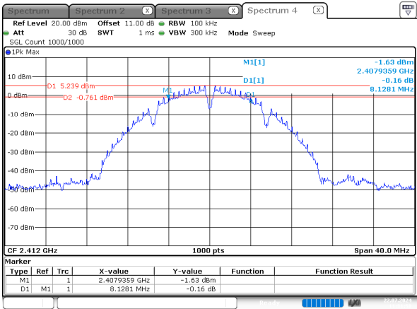
b_2412MHz_Chain 0
