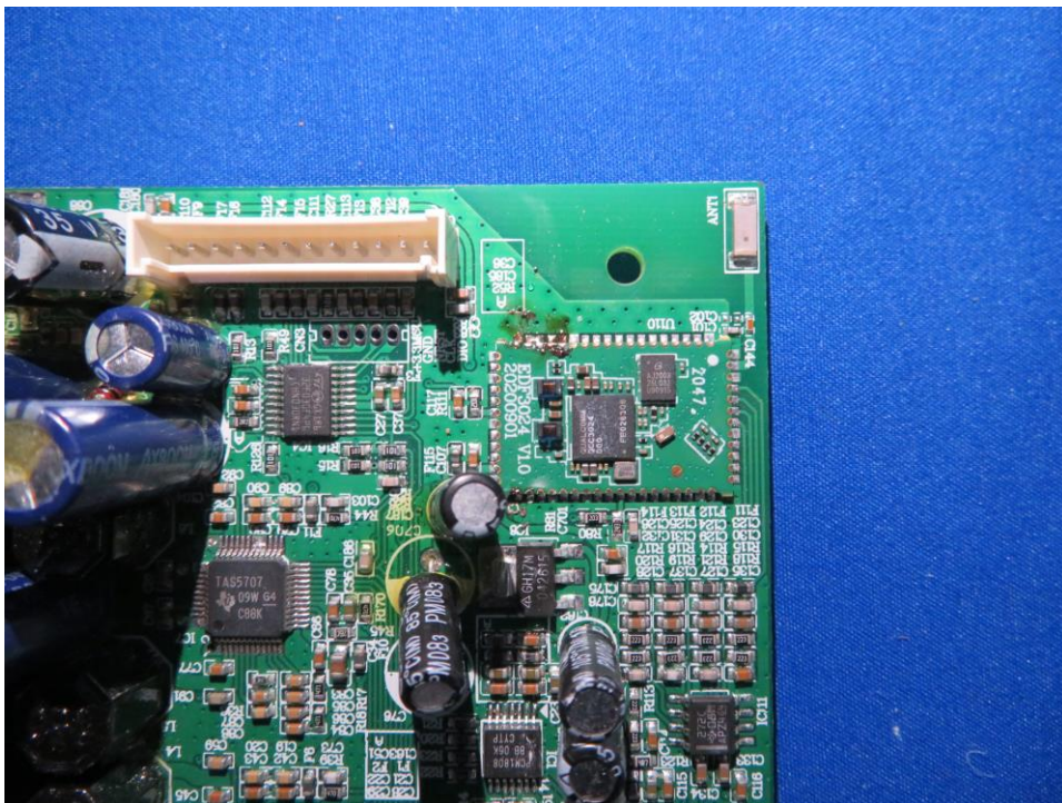
(6) EUT Photo
