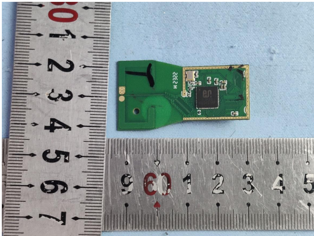
2.4G ANT
