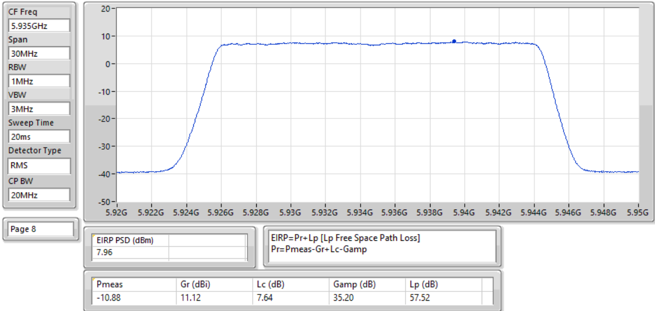
EIRP PSD;Band:6.2G;QPSK;BWch:20MHz;Nss:1;Nant:2;Ch:5935MHz;TX
