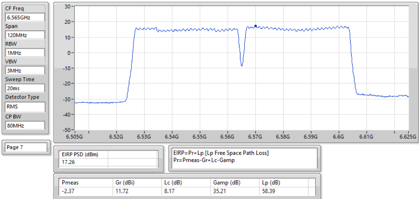
EIRP PSD;Band:6.7G;QPSK40+40 ;BWch:80MHz;Nss:1;Nant:2;Ch:#6545,#6585MHz;TX
