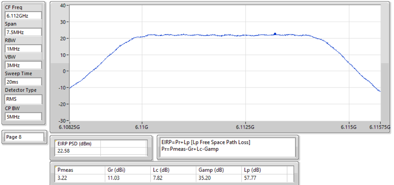
EIRP PSD;Band:6.2G;QPSK;BWch:5MHz;Nss:1;Nant:2;Ch:6112MHz;TX
