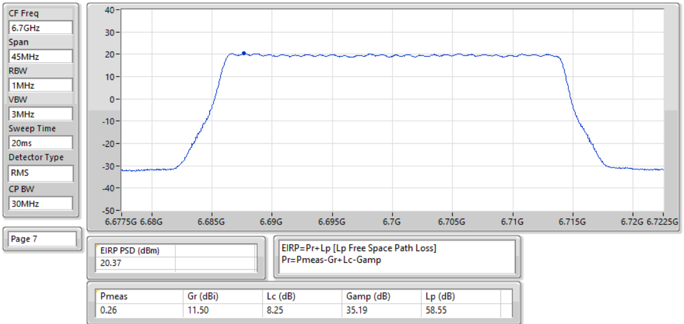
EIRP PSD;Band:6.7G;QPSK;BWch:30MHz;Nss:1;Nant:2;Ch:6700MHz;TX
