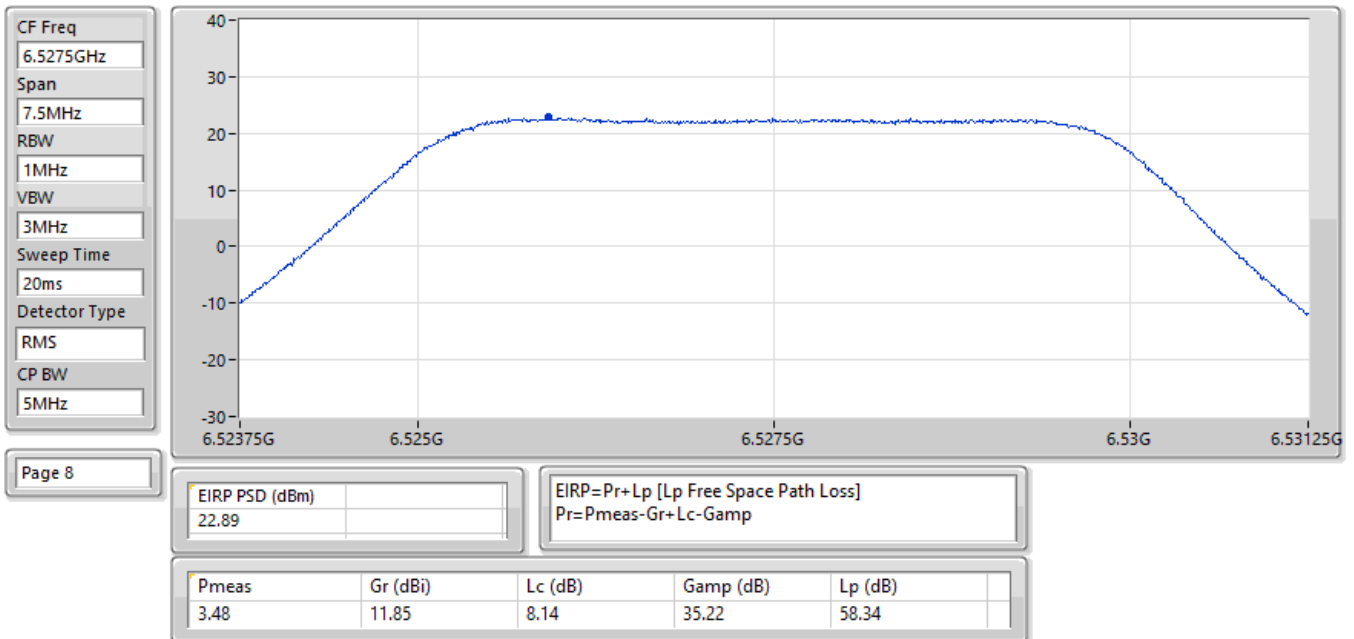
EIRP PSD;Band:6.7G;QPSK;BWch:5MHz;Nss:1;Nant:2;Ch:6527.5MHz;TX
