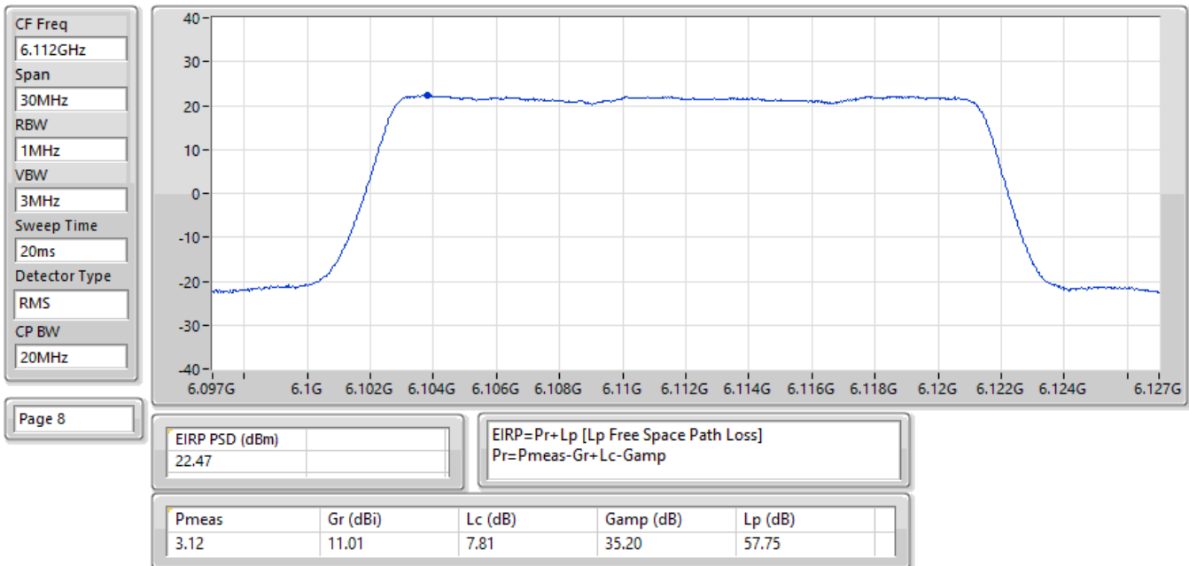
EIRP PSD;Band:6.2G;QPSK;BWch:20MHz;Nss:1;Nant:2;Ch:6112MHz;TX
