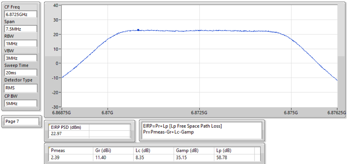
EIRP PSD;Band:6.7G;QPSK;BWch:5MHz;Nss:1;Nant:2;Ch:6872.5MHz;TX
