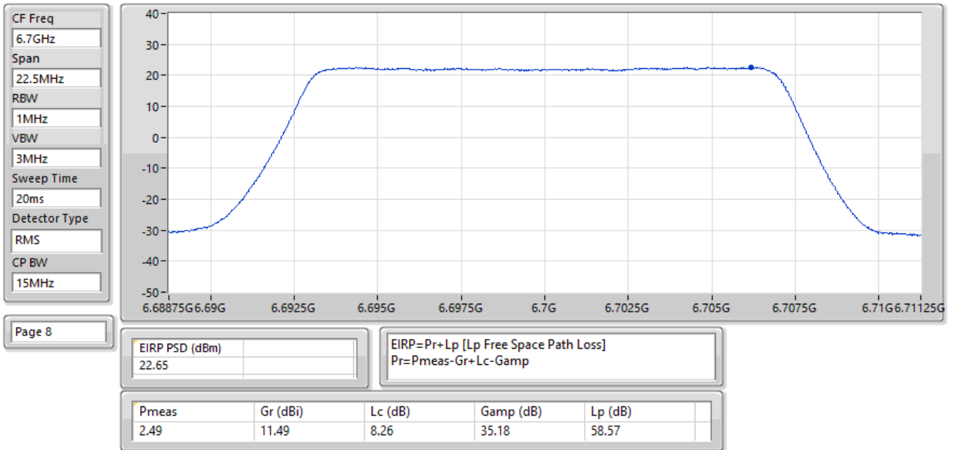
EIRP PSD;Band:6.7G;QPSK;BWch:15MHz;Nss:1;Nant:2;Ch:6700MHz;TX
