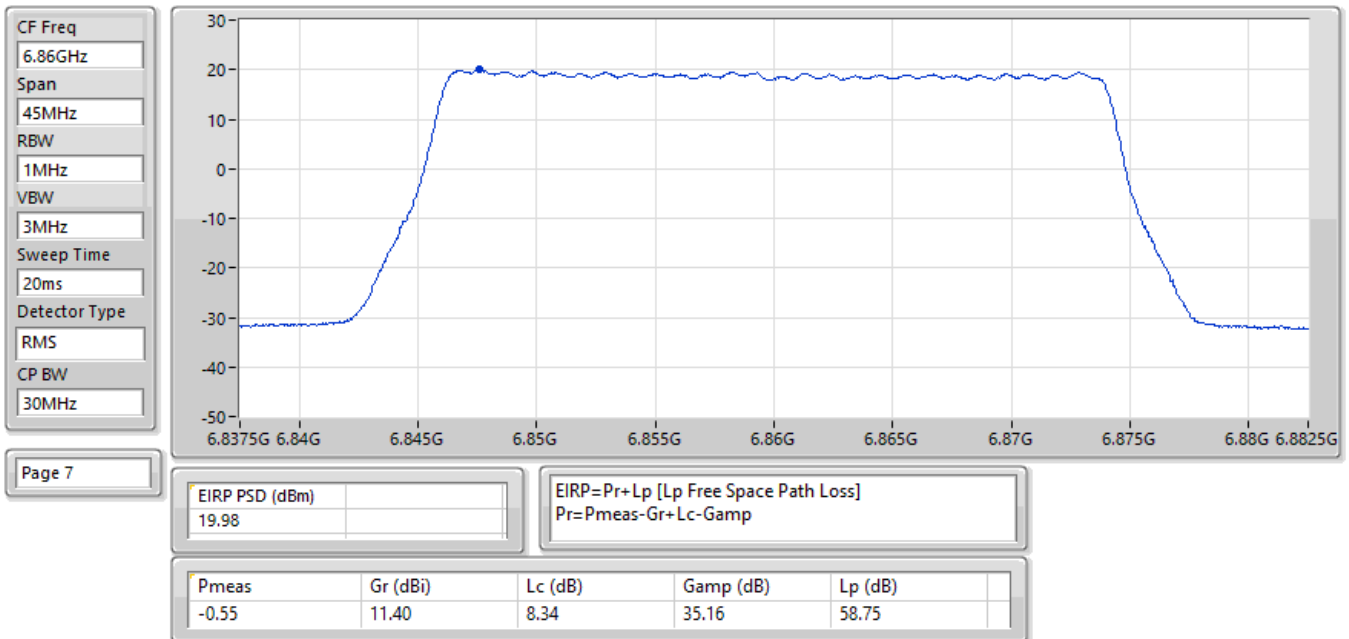
EIRP PSD;Band:6.7G;QPSK;BWch:30MHz;Nss:1;Nant:2;Ch:6860MHz;TX
