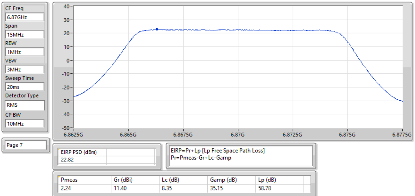
EIRP PSD;Band:6.7G;QPSK;BWch:10MHz;Nss:1;Nant:2;Ch:6870MHz;TX
