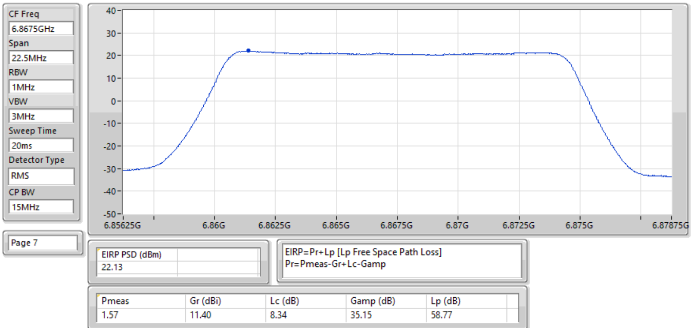
EIRP PSD;Band:6.7G;QPSK;BWch:15MHz;Nss:1;Nant:2;Ch:6867.5MHz;TX
