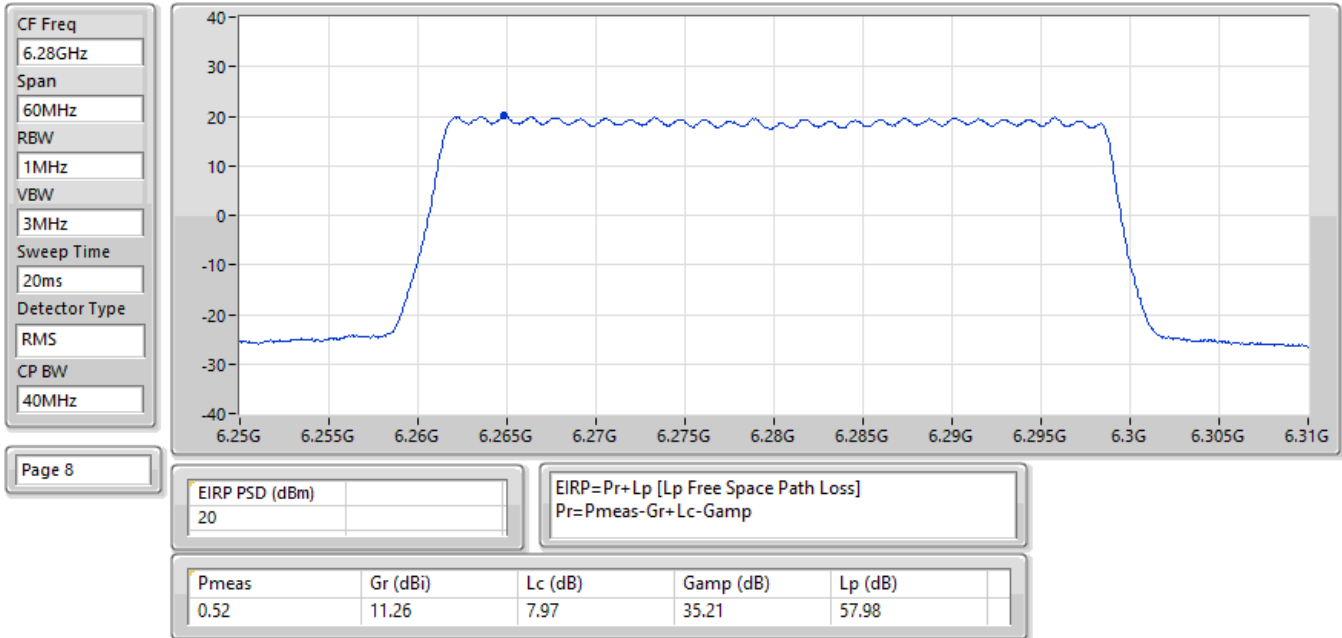
EIRP PSD;Band:6.2G;QPSK;BWch:40MHz;Nss:1;Nant:2;Ch:6280MHz;TX
