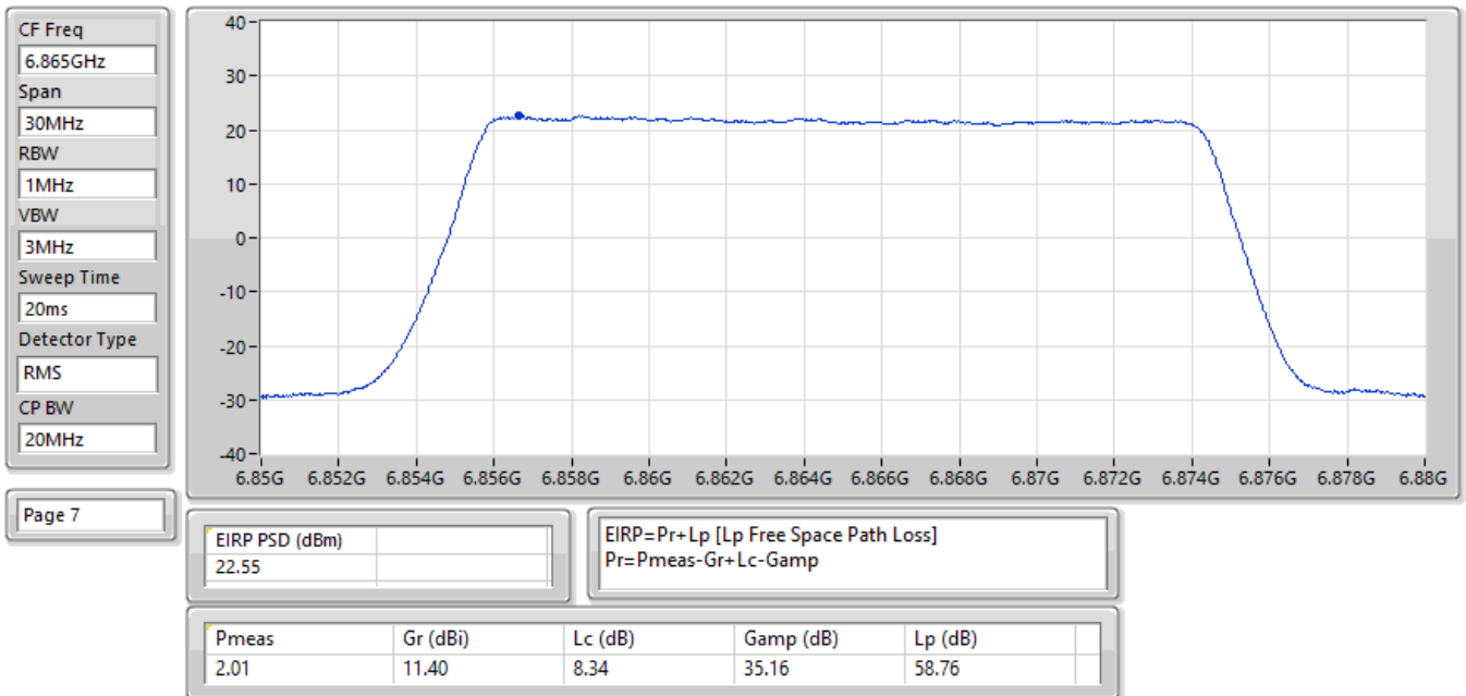
EIRP PSD;Band:6.7G;QPSK;BWch:20MHz;Nss:1;Nant:2;Ch:6865MHz;TX
