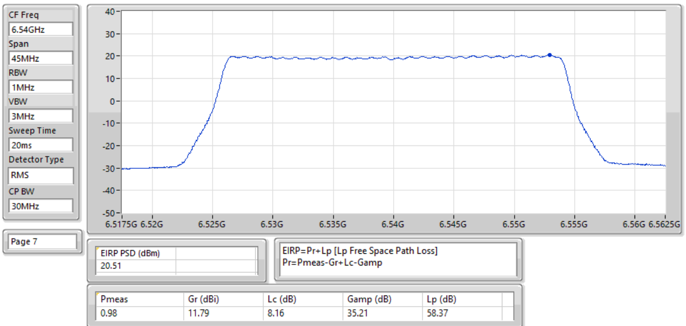
EIRP PSD;Band:6.7G;QPSK;BWch:30MHz;Nss:1;Nant:2;Ch:6540MHz;TX
