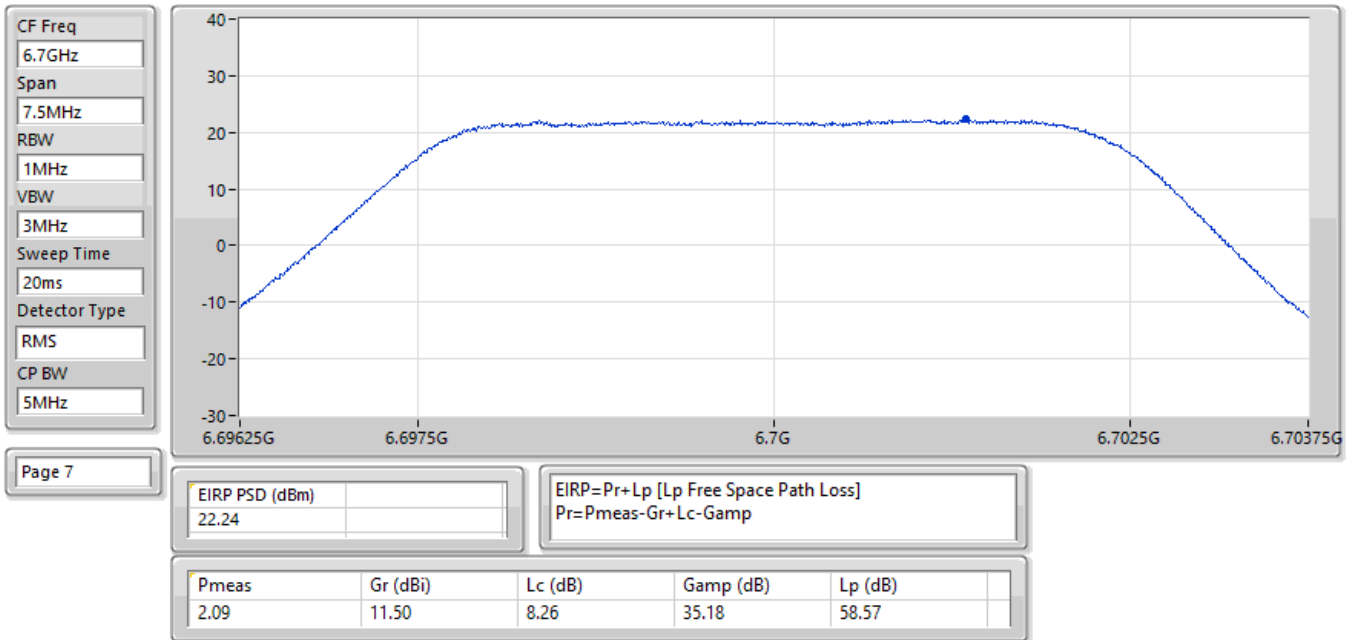
EIRP PSD;Band:6.7G;QPSK;BWch:5MHz;Nss:1;Nant:2;Ch:6700MHz;TX
