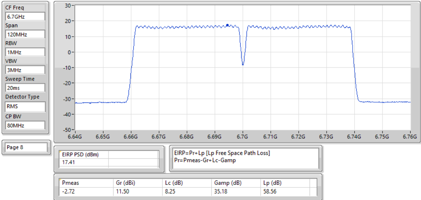
EIRP PSD;Band:6.7G;QPSK40+40 ;BWch:80MHz;Nss:1;Nant:2;Ch:#6680,#6720MHz;TX
