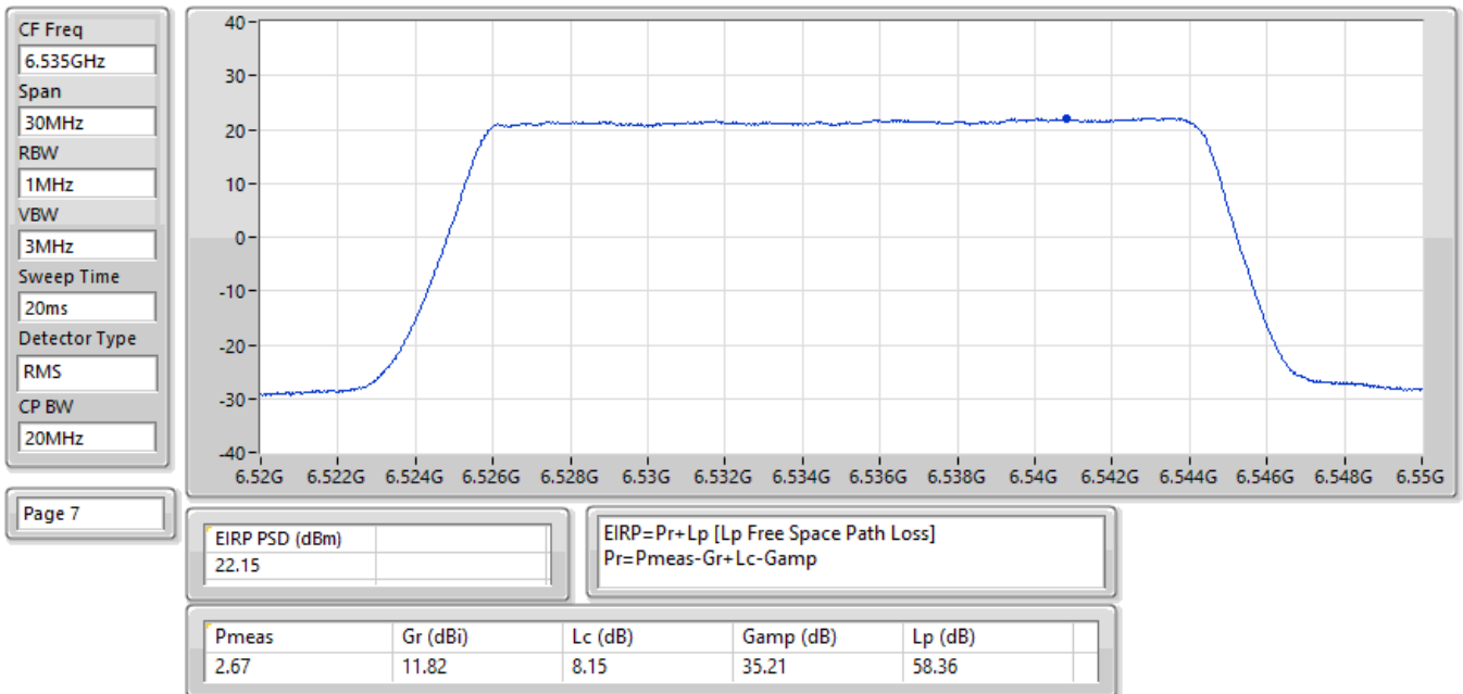
EIRP PSD;Band:6.7G;QPSK;BWch:20MHz;Nss:1;Nant:2;Ch:6535MHz;TX
