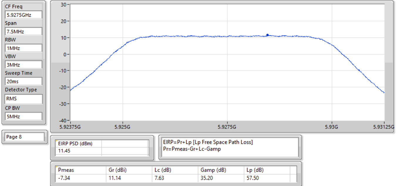
EIRP PSD;Band:6.2G;QPSK;BWch:5MHz;Nss:1;Nant:2;Ch:5927.5MHz;TX
