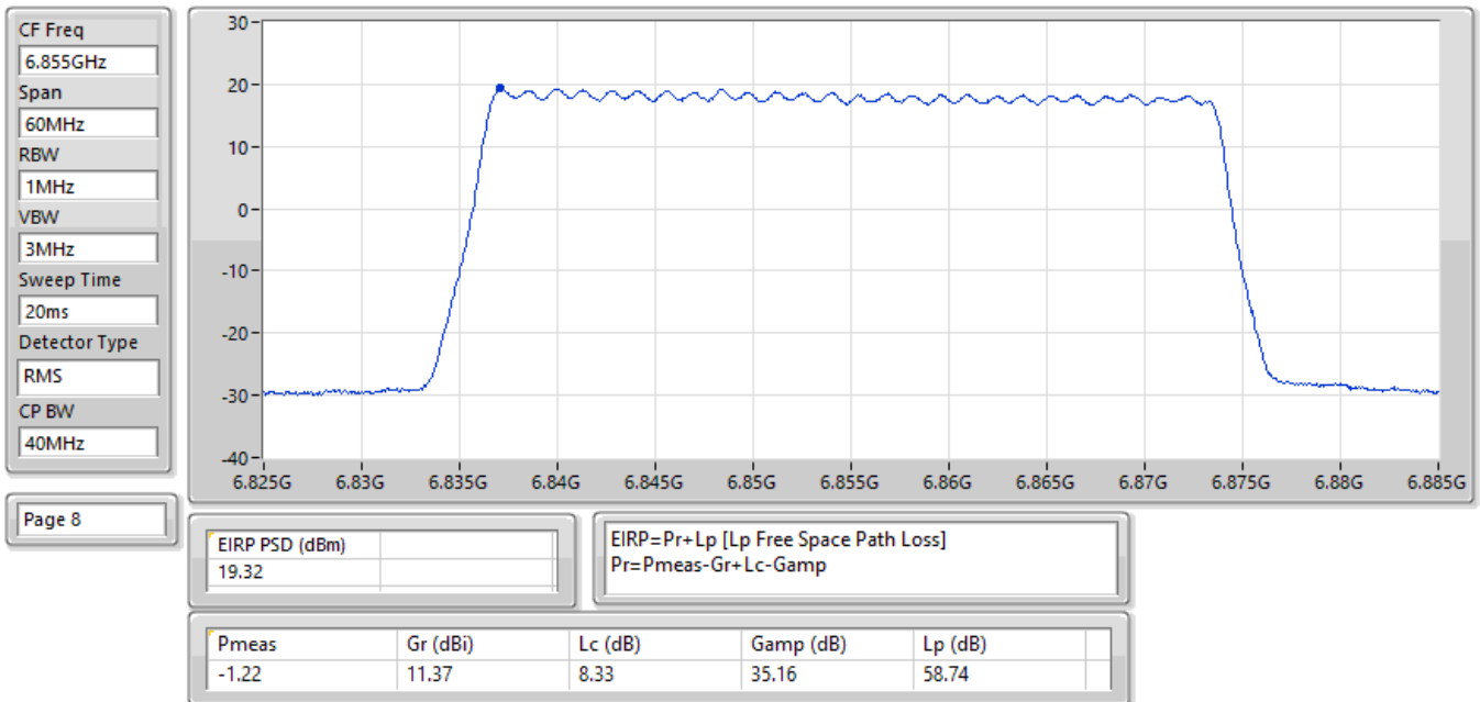
EIRP PSD;Band:6.7G;QPSK;BWch:40MHz;Nss:1;Nant:2;Ch:6855MHz;TX
