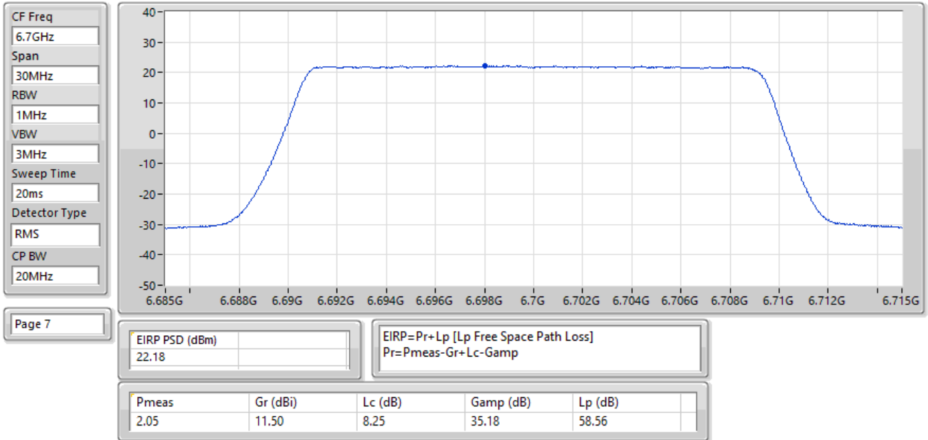
EIRP PSD;Band:6.7G;QPSK;BWch:20MHz;Nss:1;Nant:2;Ch:6700MHz;TX
