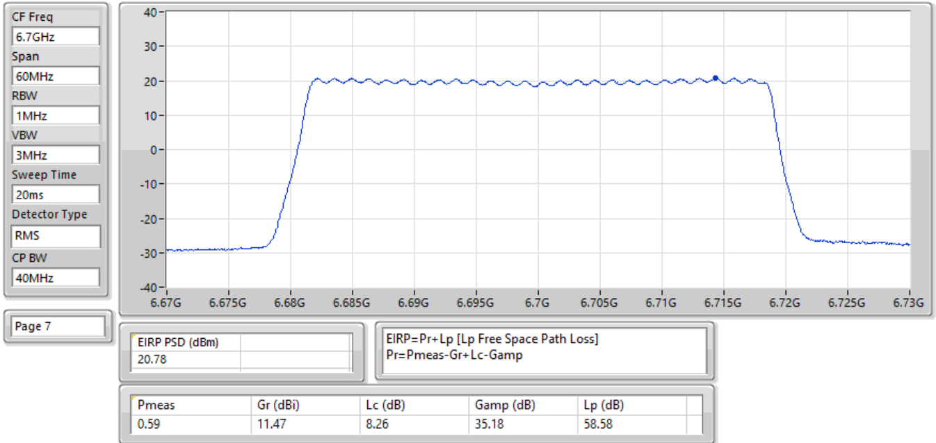
EIRP PSD;Band:6.7G;QPSK;BWch:40MHz;Nss:1;Nant:2;Ch:6700MHz;TX
