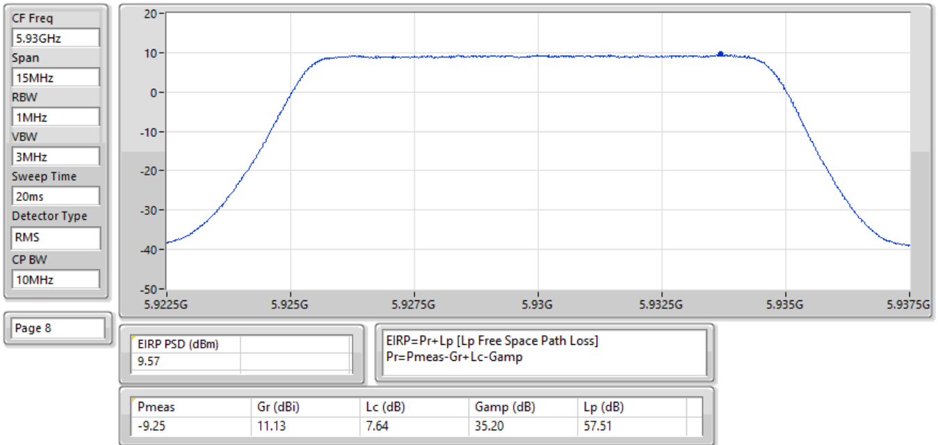
EIRP PSD;Band:6.2G;QPSK;BWch:10MHz;Nss:1;Nant:2;Ch:5930MHz;TX
