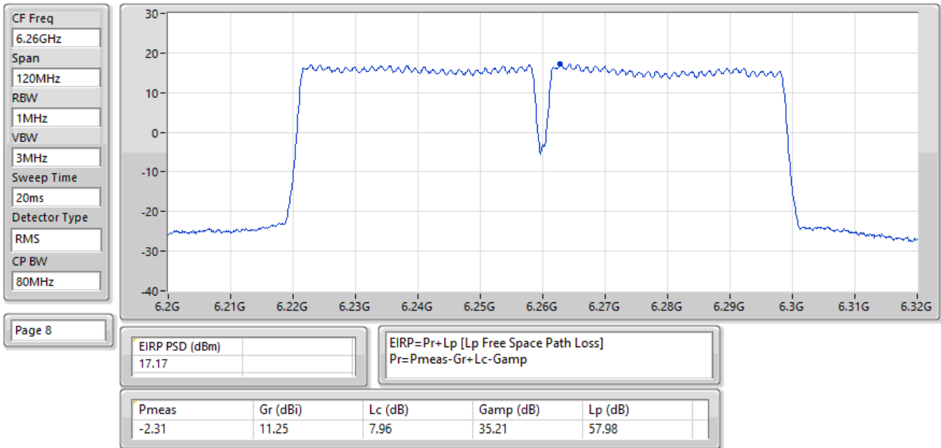
EIRP PSD;Band:6.2G;QPSK40+40 ;BWch:80MHz;Nss:1;Nant:2;Ch:#6240,#6280MHz;TX
