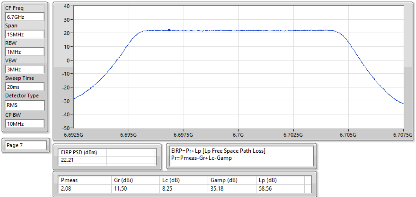
EIRP PSD;Band:6.7G;QPSK;BWch:10MHz;Nss:1;Nant:2;Ch:6700MHz;TX
