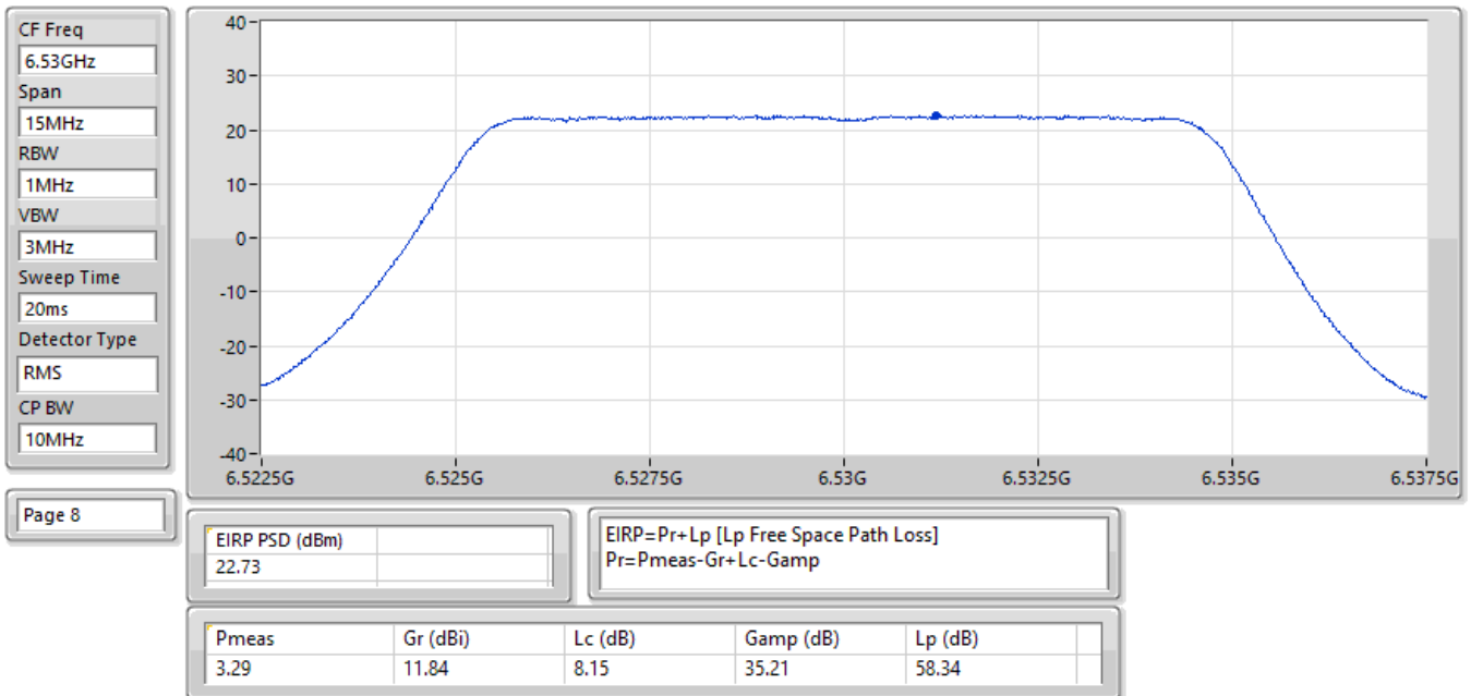
EIRP PSD;Band:6.7G;QPSK;BWch:10MHz;Nss:1;Nant:2;Ch:6530MHz;TX
