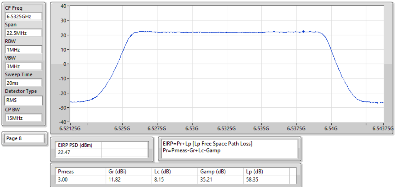
EIRP PSD;Band:6.7G;QPSK;BWch:15MHz;Nss:1;Nant:2;Ch:6532.5MHz;TX
