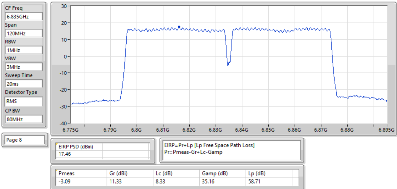
EIRP PSD;Band:6.7G;QPSK40+40 ;BWch:80MHz;Nss:1;Nant:2;Ch:#6815,#6855MHz;TX
