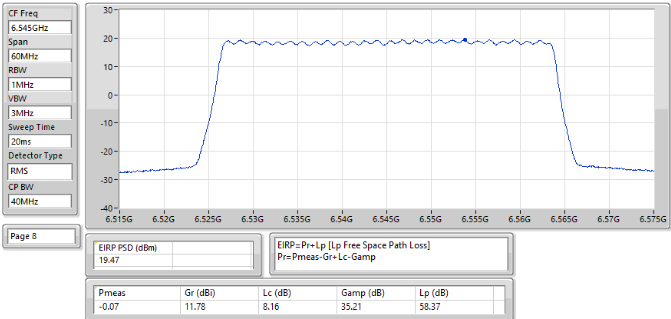
EIRP PSD;Band:6.7G;QPSK;BWch:40MHz;Nss:1;Nant:2;Ch:6545MHz;TX
