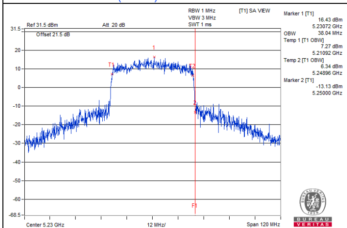
802.11ax (HE40) CDD / Chain 2 : CH 46
