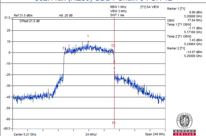
802.11ax (HE80) CDD / Chain 2 : CH 42
