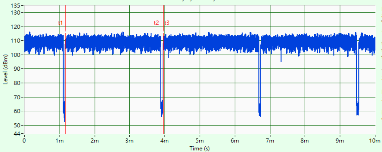
802.11ax (HE80) CDD
