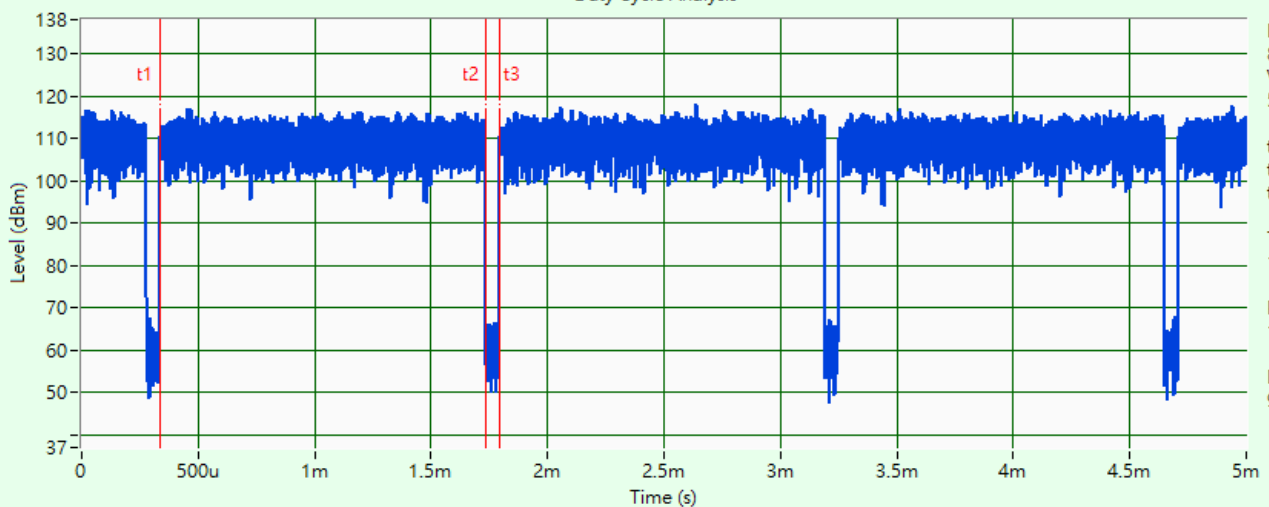
802.11ax (HE160) CDD
