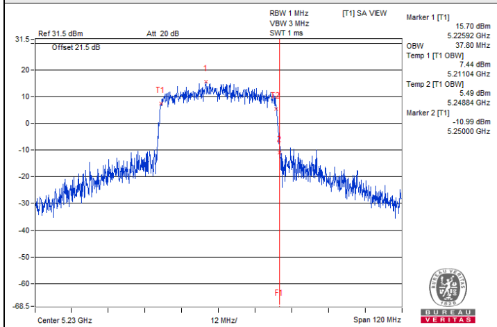
802.11ax (HE40) CDD / Chain 0 : CH 46
