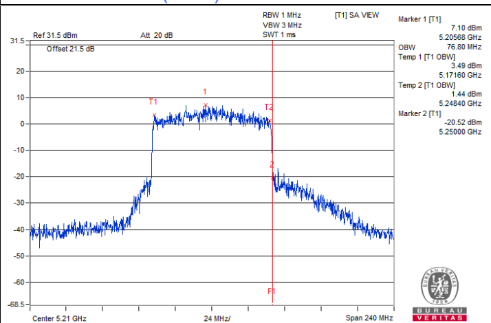
802.11ax (HE80) CDD / Chain 0 : CH 42
