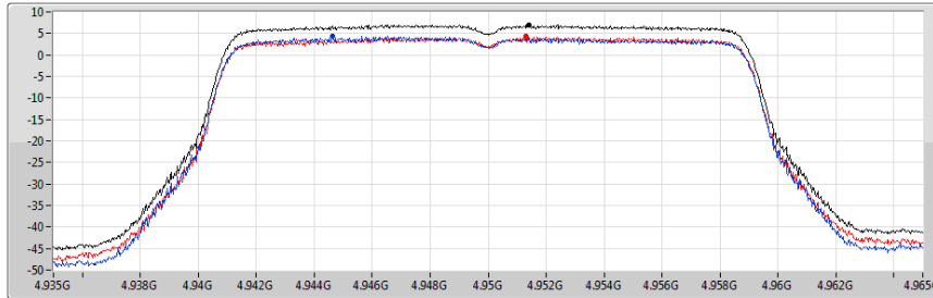
4.94-4.99GHz_802.11j_20MHz_Nss1_2TX 4950MHz
