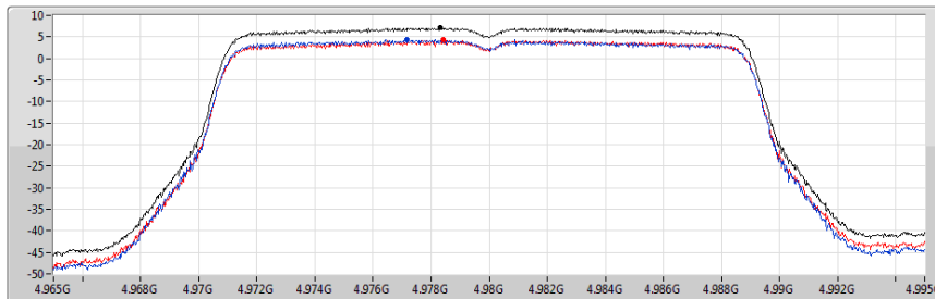
4.94-4.99GHz_802.11j_20MHz_Nss1_2TX 4980MHz
