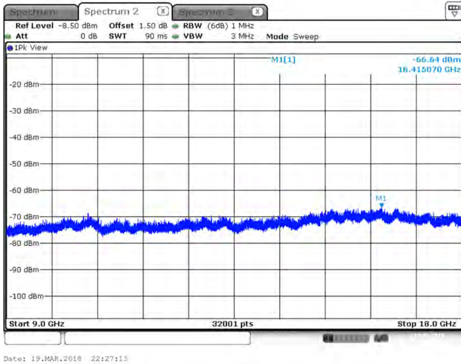
Plot on IEEE 802.11ac Nss1 MCS0 VHT80 / 5690 MHz / Peak / Port 2 / 9GHz~18GHz
