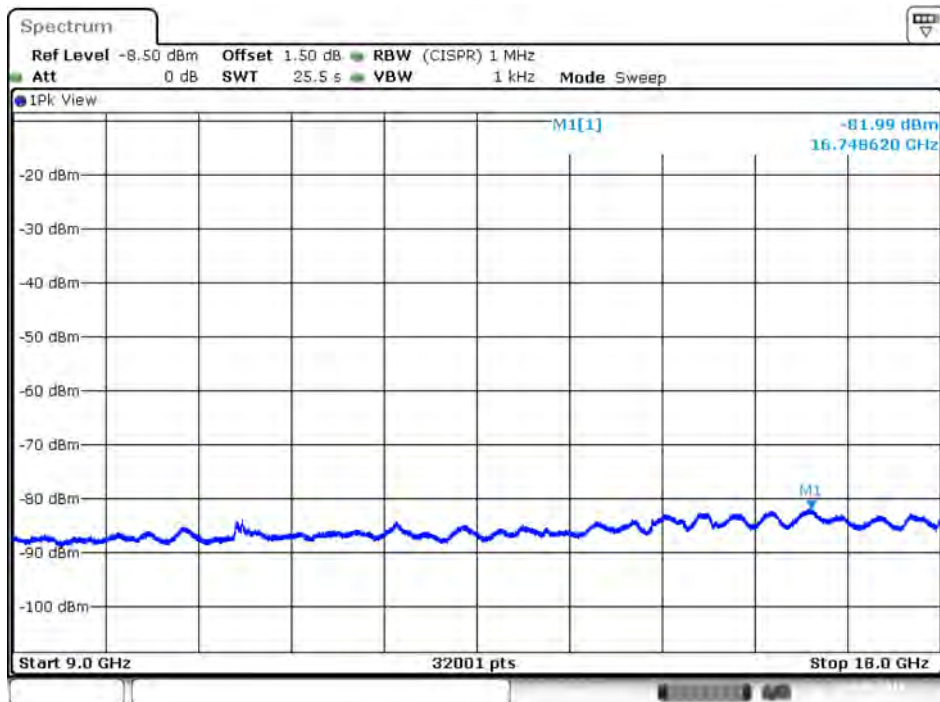
Plot on IEEE 802.11ac Nss1 MCS0 VHT80 / 5610 MHz / Average / Port 1 / 9GHz~18GHz
