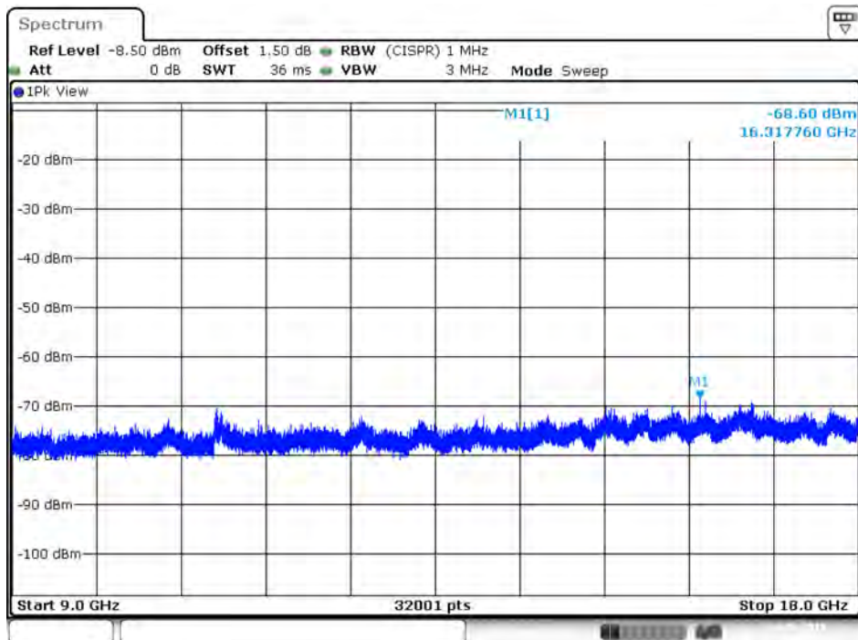
Plot on IEEE 802.11ac Nss1 MCS0 VHT80 / 5610 MHz / Peak / Port 1 / 9GHz~18GHz
