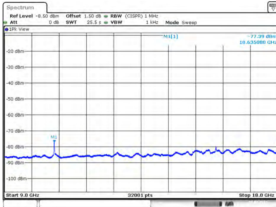
Plot on IEEE 802.11ac Nss1 MCS0 VHT20 / 5320 MHz / Average / Port 1 / 9GHz~18GHz
