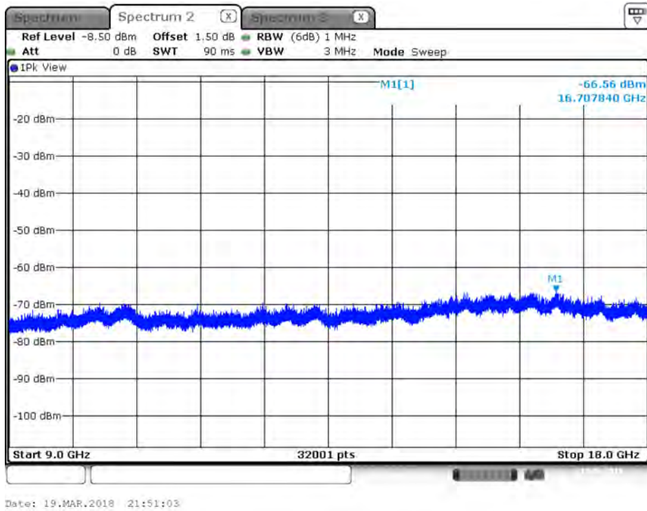
Plot on IEEE 802.11ac Nss1 MCS0 VHT80 / 5610 MHz / Peak / Port 1 / 9GHz~18GHz
