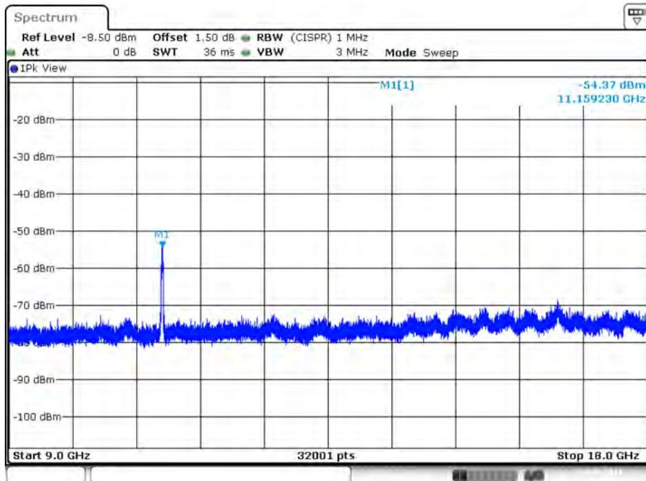
Plot on IEEE 802.11ac Nss1 MCS0 VHT20 / 5580 MHz / Peak / Port 1 / 9GHz~18GHz
