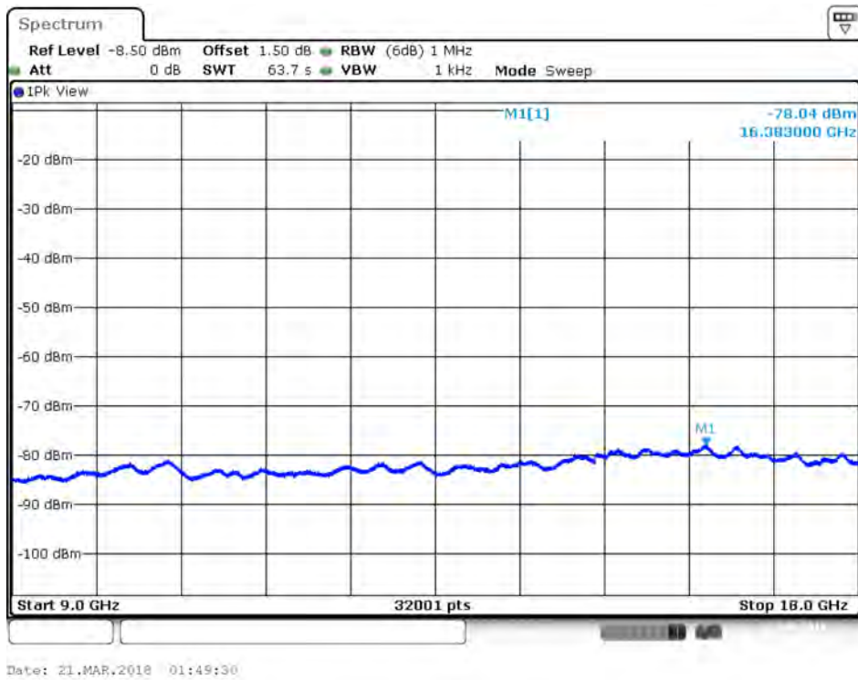
Plot on IEEE 802.11ac Nss1 MCS0 VHT80 / 5290 MHz / Peak / Port 1 / 9GHz~18GHz
