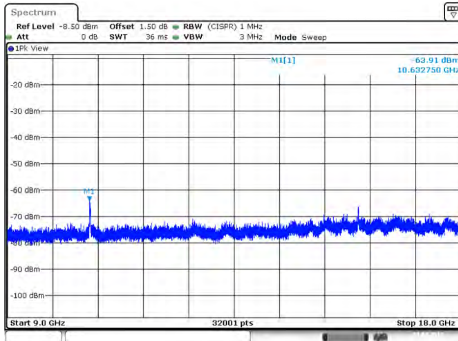
Plot on IEEE 802.11ac Nss1 MCS0 VHT20 / 5320 MHz / Peak / Port 1 / 9GHz~18GHz
