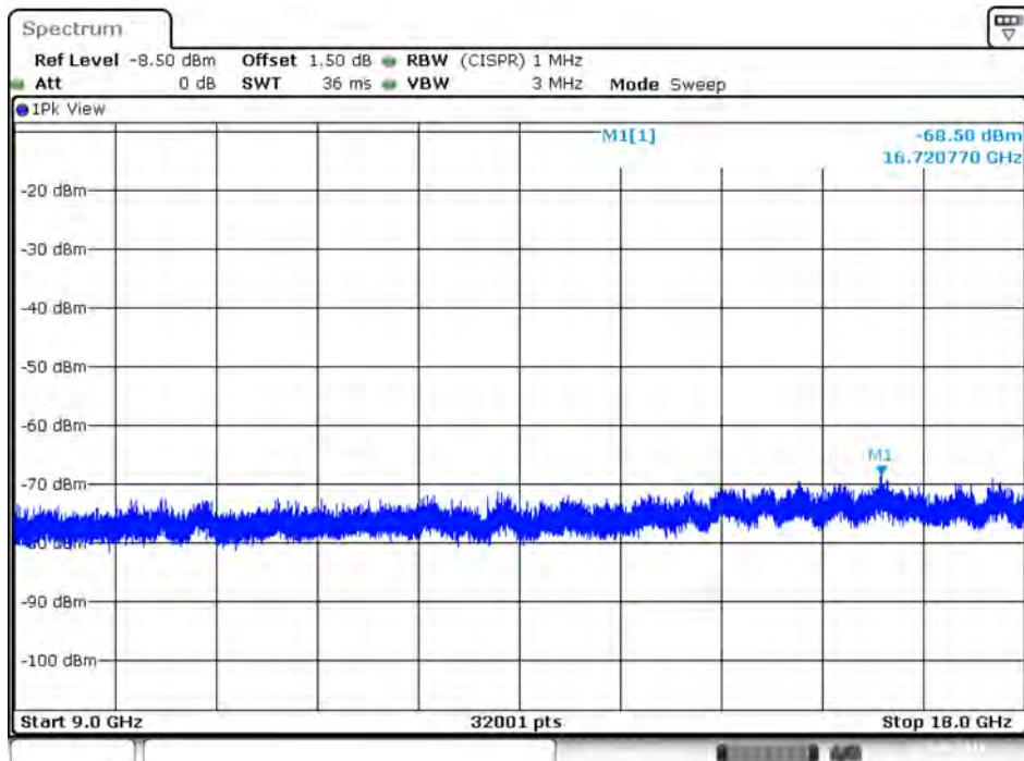
Plot on IEEE 802.11ac Nss1 MCS0 VHT80 / 5290 MHz / Peak / Port 1 / 9GHz~18GHz
