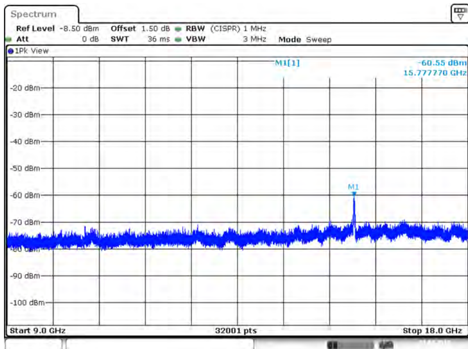
Plot on IEEE 802.11ac Nss1 MCS0 VHT20 / 5260 MHz / Peak / Port 1 / 9GHz~18GHz
