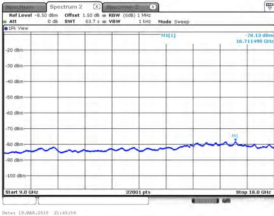
Plot on IEEE 802.11ac Nss1 MCS0 VHT80 / 5530 MHz / Peak / Port 2 / 9GHz~18GHz
