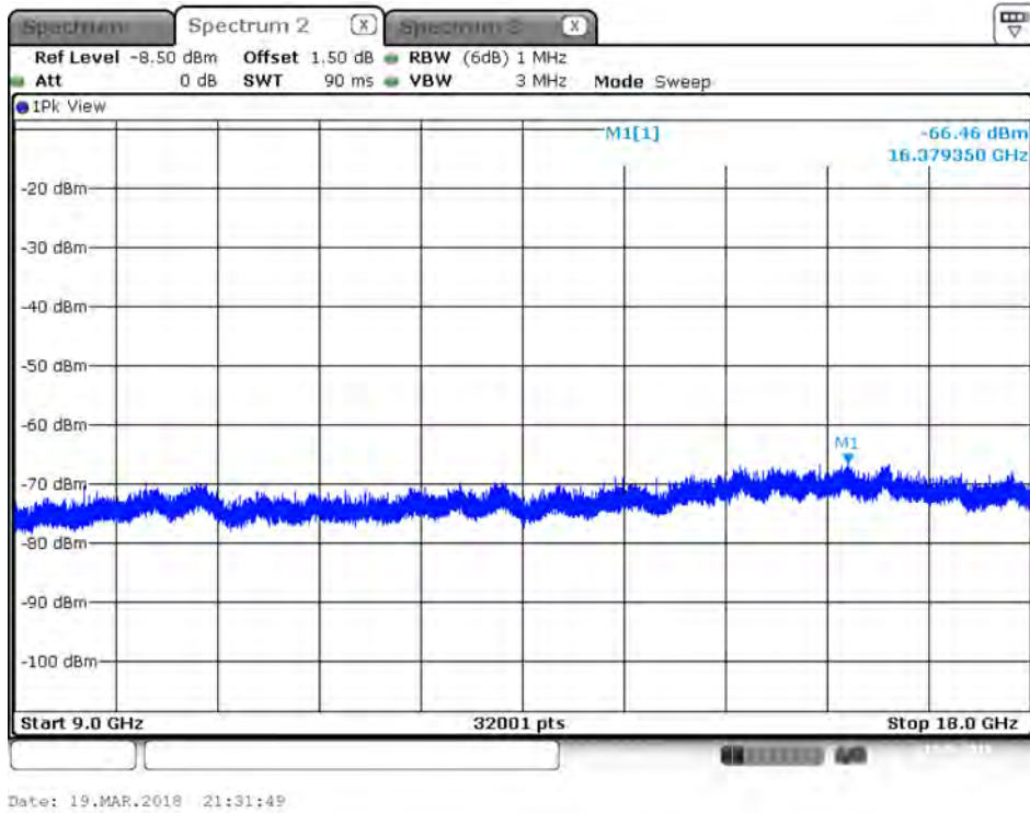
Plot on IEEE 802.11ac Nss1 MCS0 VHT80 / 5530 MHz / Peak / Port 1 / 9GHz~18GHz
