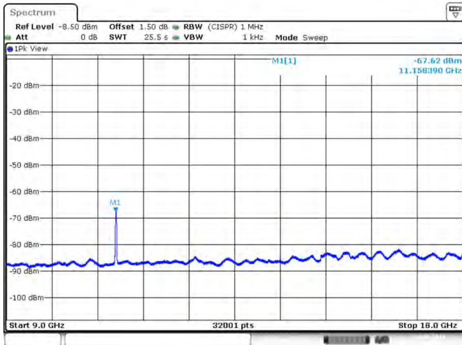
Plot on IEEE 802.11ac Nss1 MCS0 VHT20 / 5580 MHz / Average / Port 1 / 9GHz~18GHz
