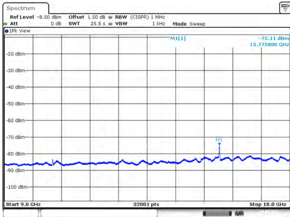
Plot on IEEE 802.11ac Nss1 MCS0 VHT20 / 5260 MHz / Average / Port 1 / 9GHz~18GHz
