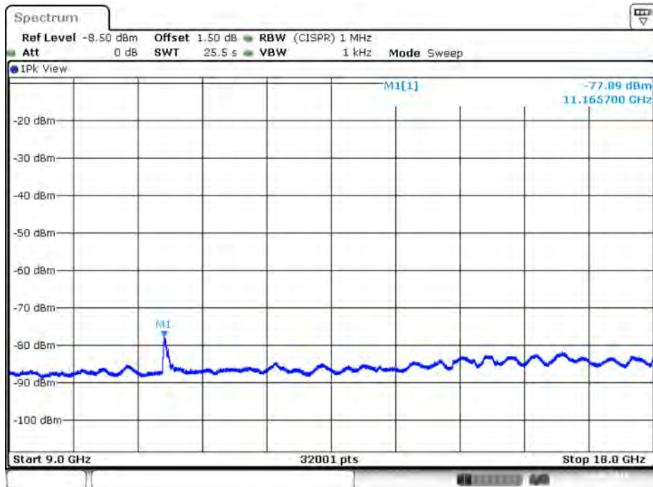
Plot on IEEE 802.11ac Nss1 MCS0 VHT80 / 5610 MHz / Average / Port 2 / 9GHz~18GHz
