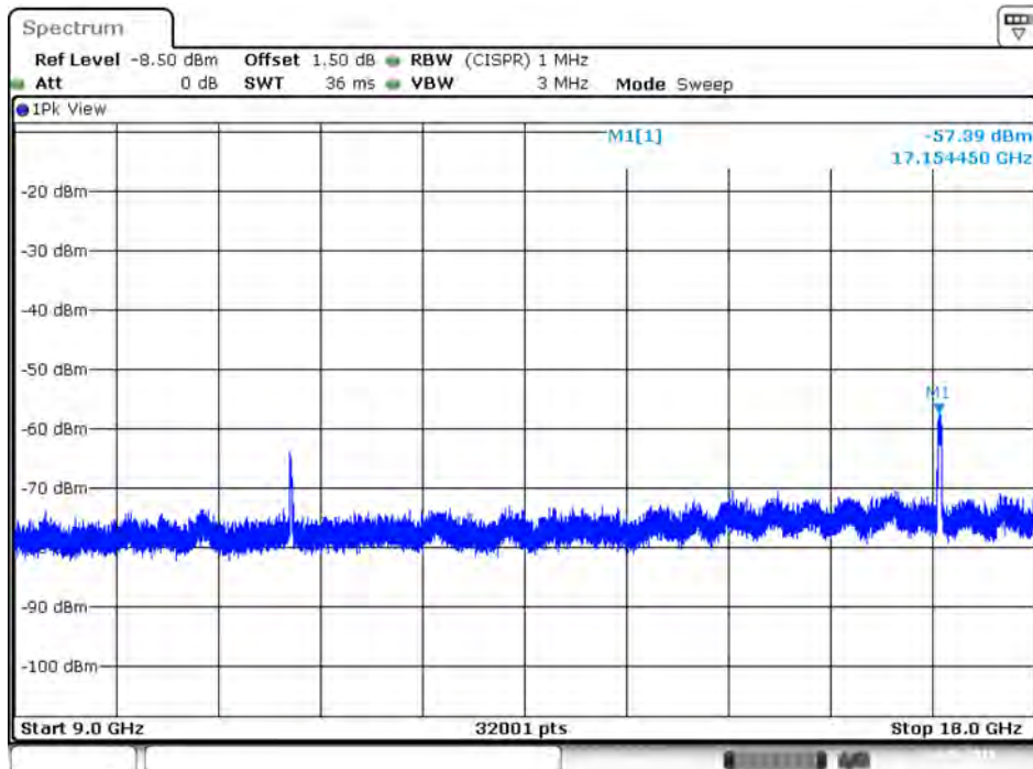
Plot on IEEE 802.11ac Nss1 MCS0 VHT20 / 5720 MHz / Peak / Port 1 / 9GHz~18GHz
