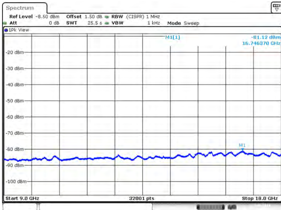
Plot on IEEE 802.11ac Nss1 MCS0 VHT80 / 5290 MHz / Average / Port 1 / 9GHz~18GHz
