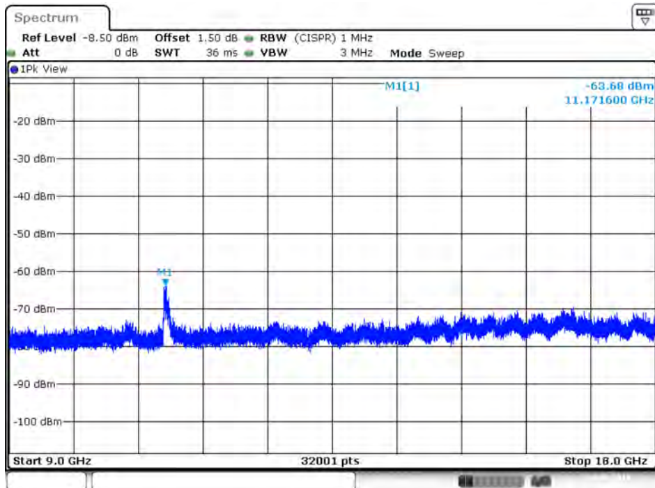
Plot on IEEE 802.11ac Nss1 MCS0 VHT80 / 5610 MHz / Peak / Port 2 / 9GHz~18GHz
