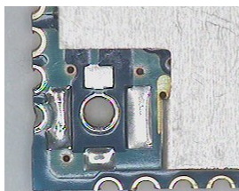
【Wire antenna】
