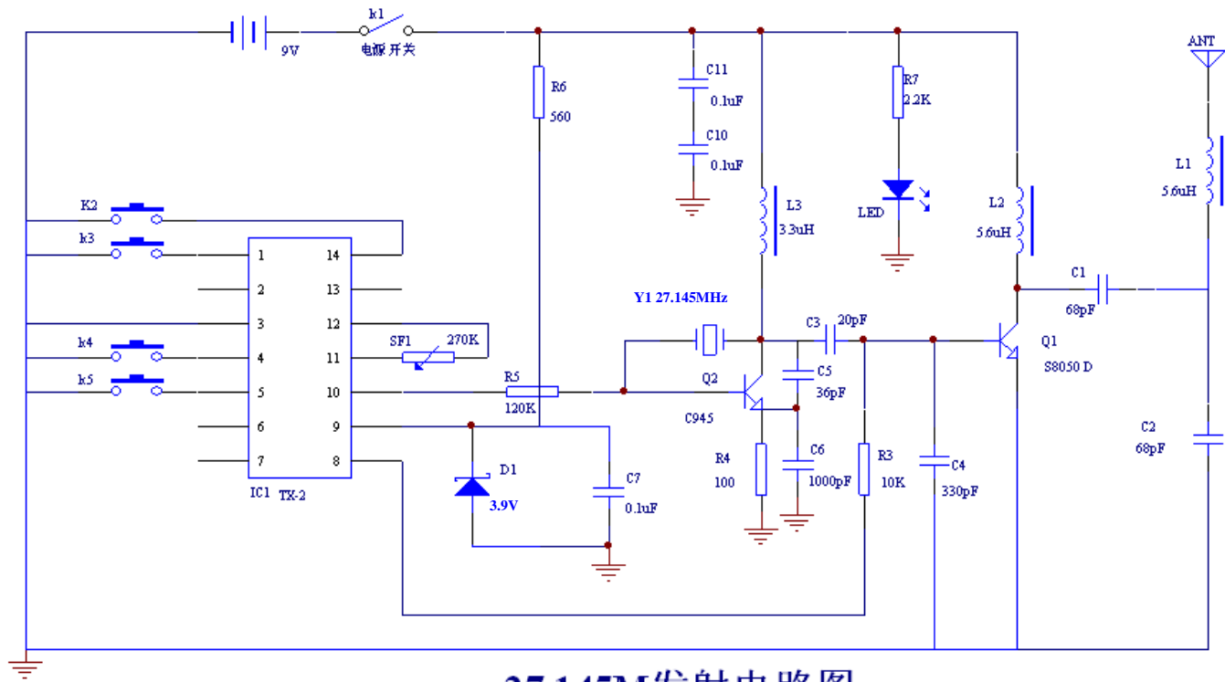
27.145M发射电路图
