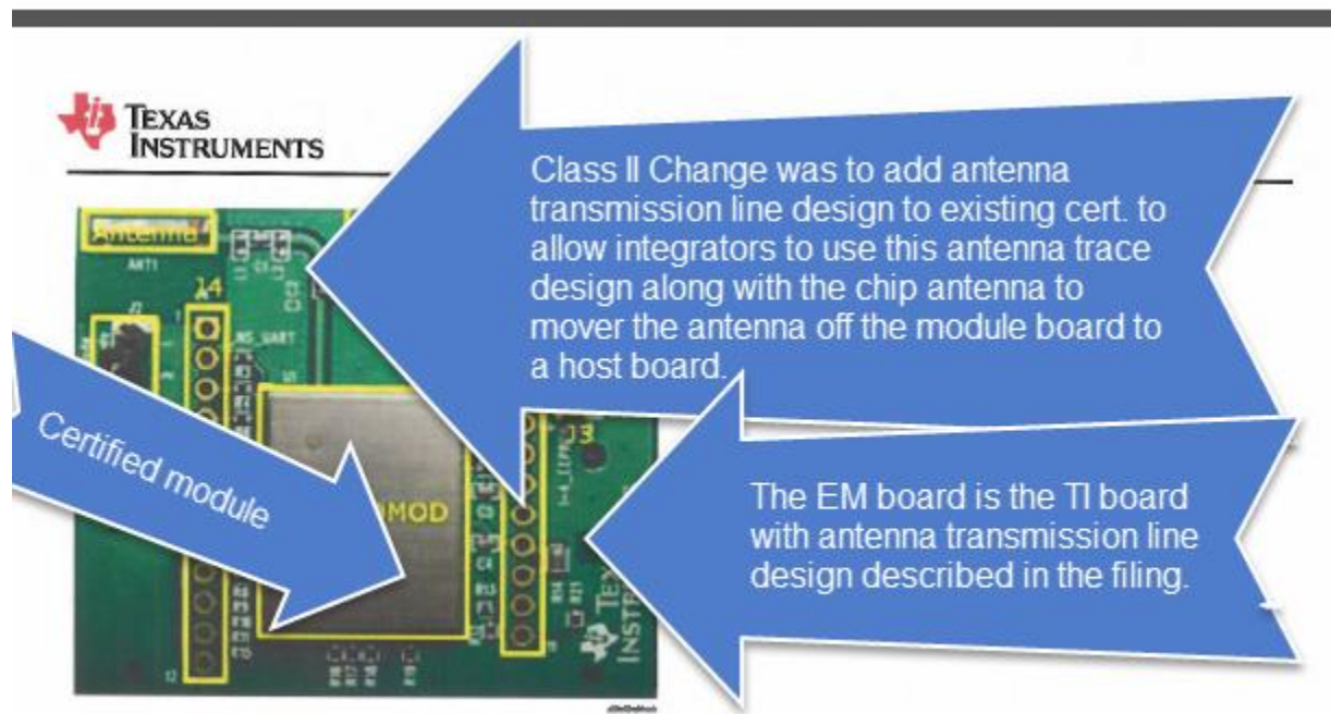
Figure 2-1. CC3000 EM Board Top View
