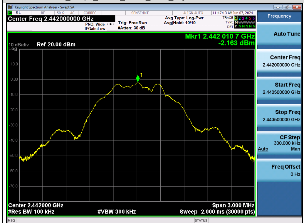
Test_Graph_GFSK_ANT1_2442_Reference Level
