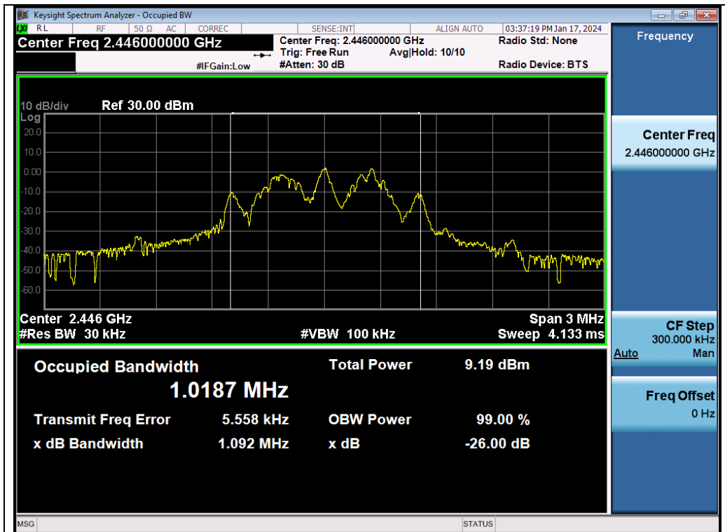
Test_Graph_GFSK_ANT1_2446_OBW
