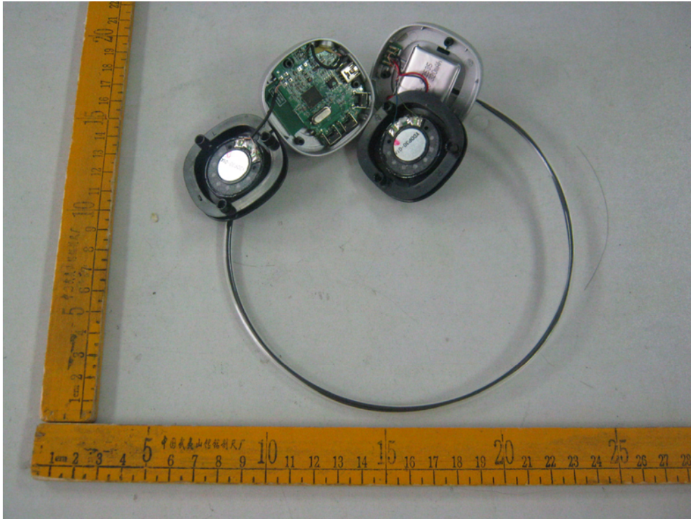
Bluetooth module
