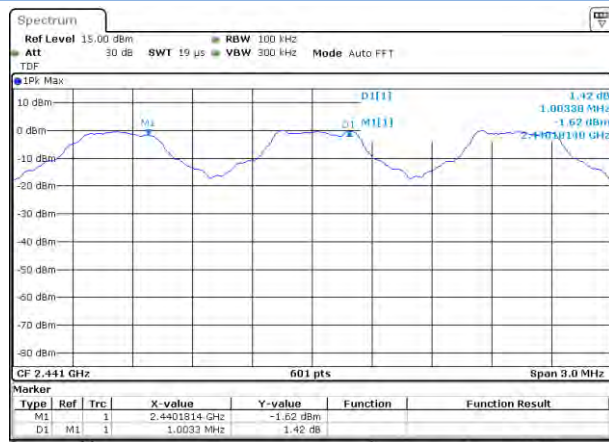
GFSK
