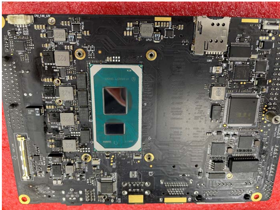
CPU-A1135
