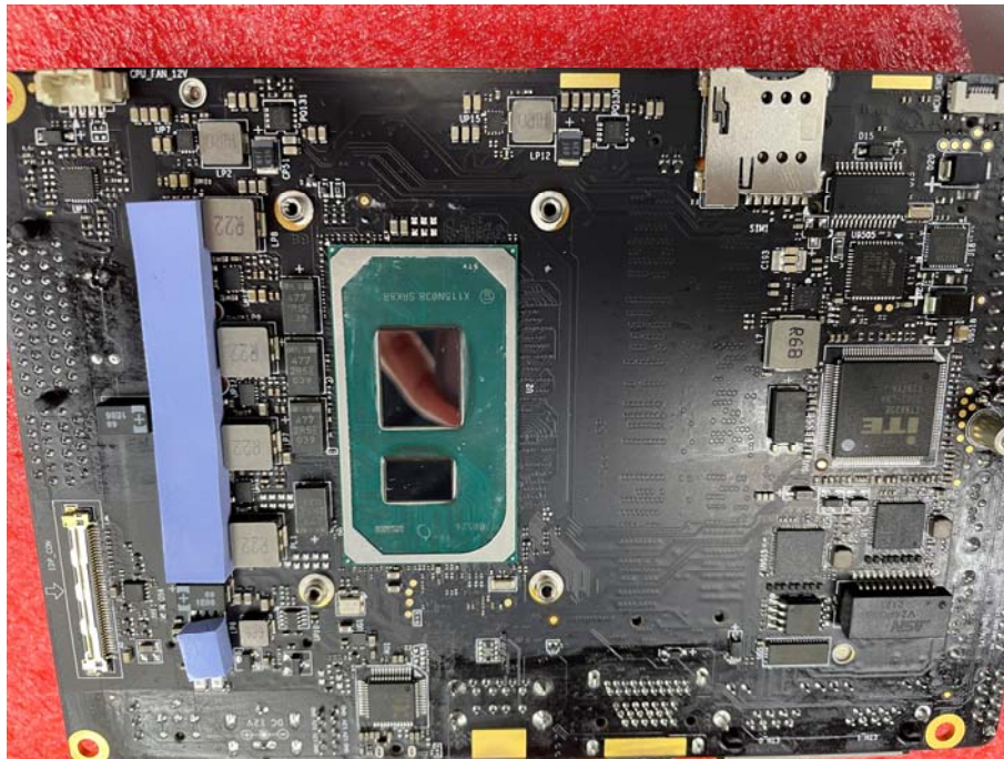
CPU-A1125
