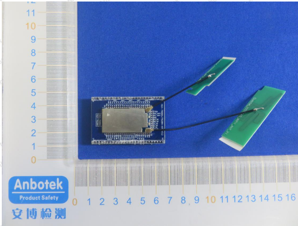
PCB ANT
