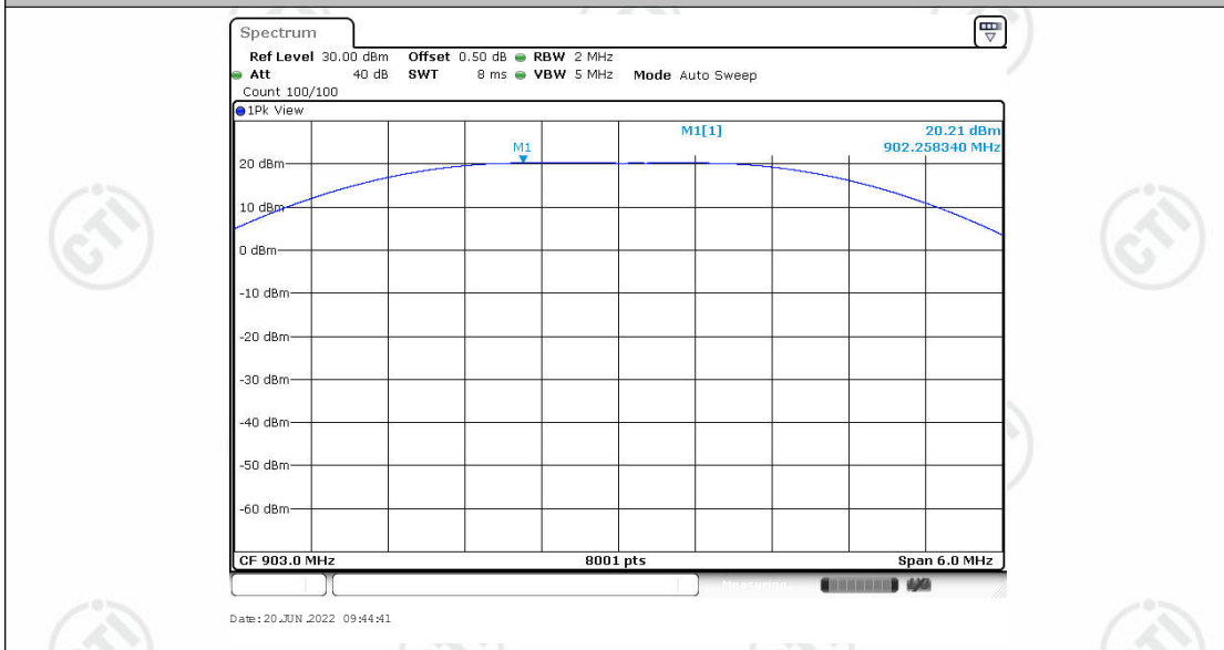
BW1523.4K_Ant1_903
