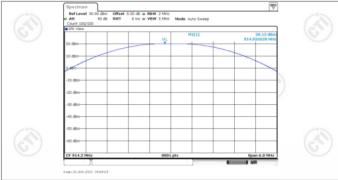
BW500K_Ant1_914.2
