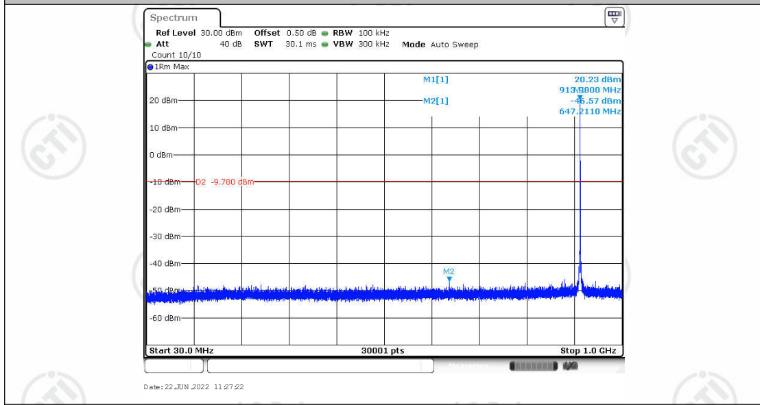
BW500K_Ant1_914.2_30~1000
