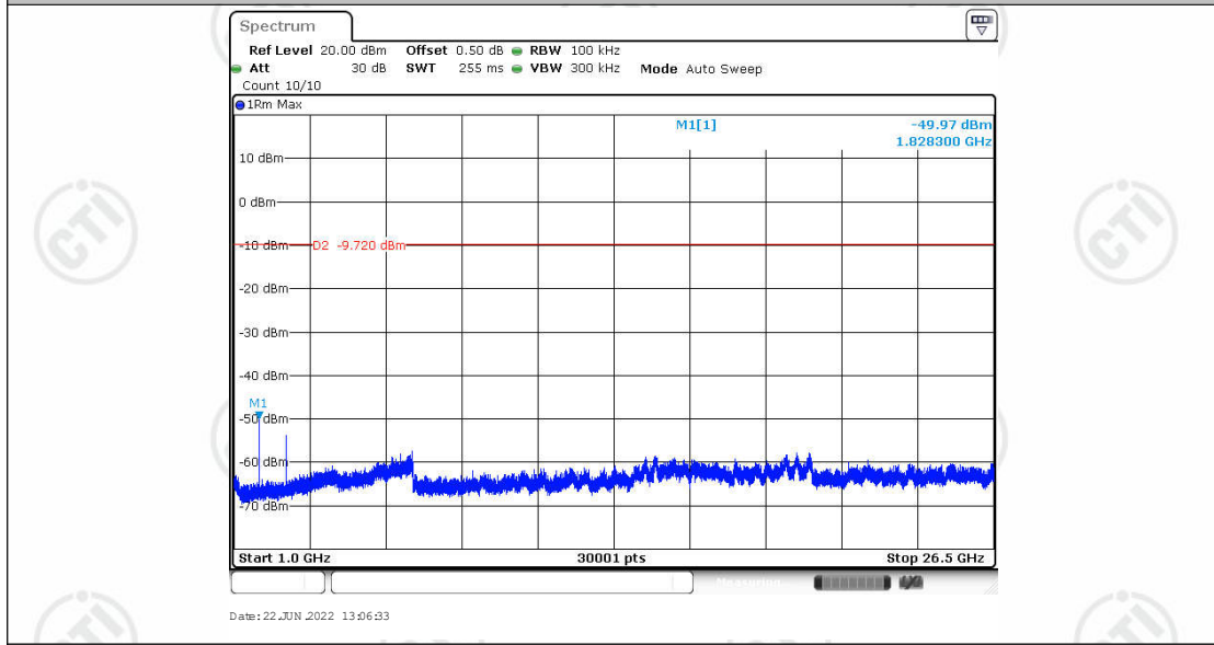
BW1523.4K_Ant1_914.2_1000~26500
