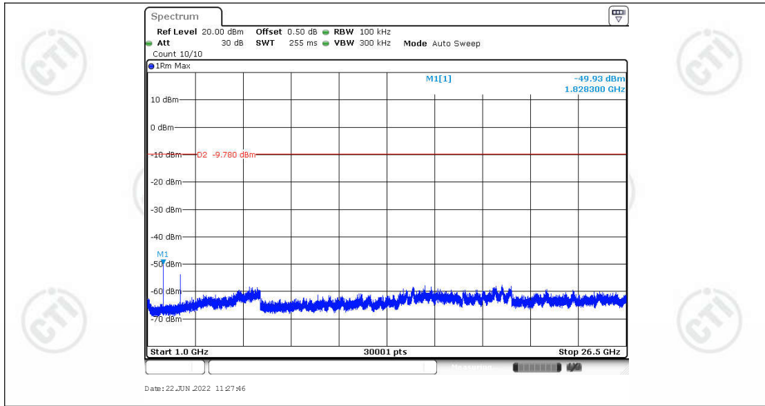
BW500K_Ant1_914.2_1000~26500
