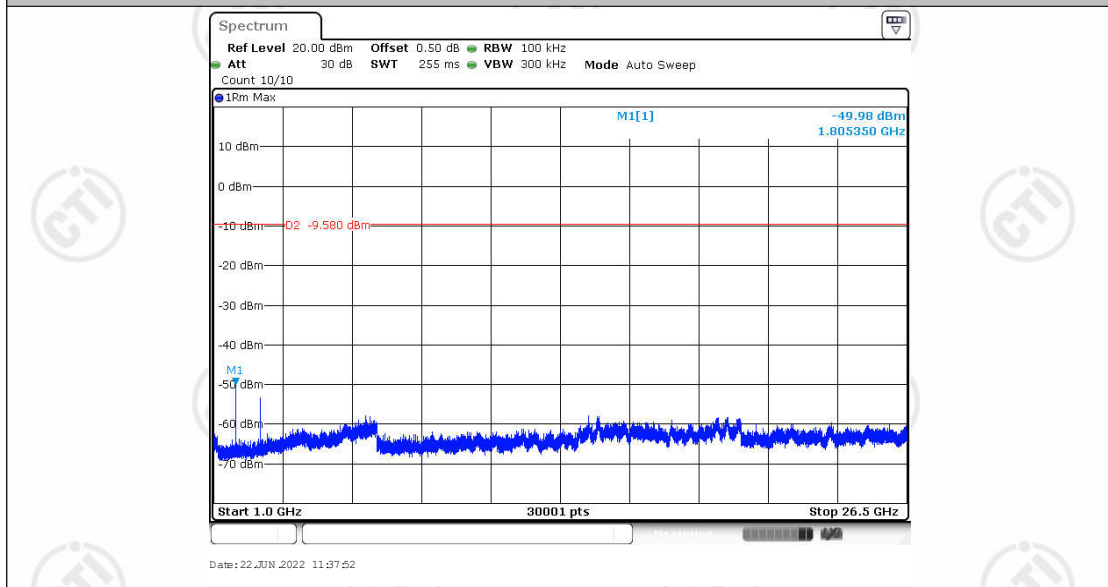
BW1523.4K_Ant1_903_1000~26500
