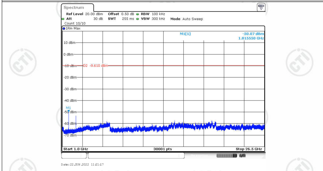
BW500K_Ant1_907.8_1000~26500
