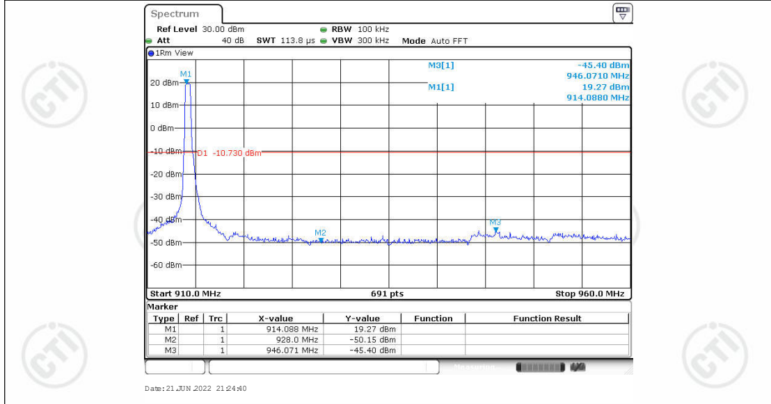
BW500K_Ant1_914.2
