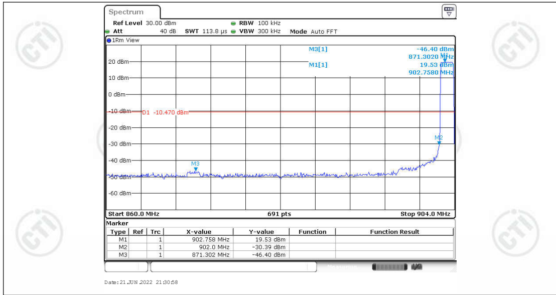
BW1523.4K_Ant1_903
