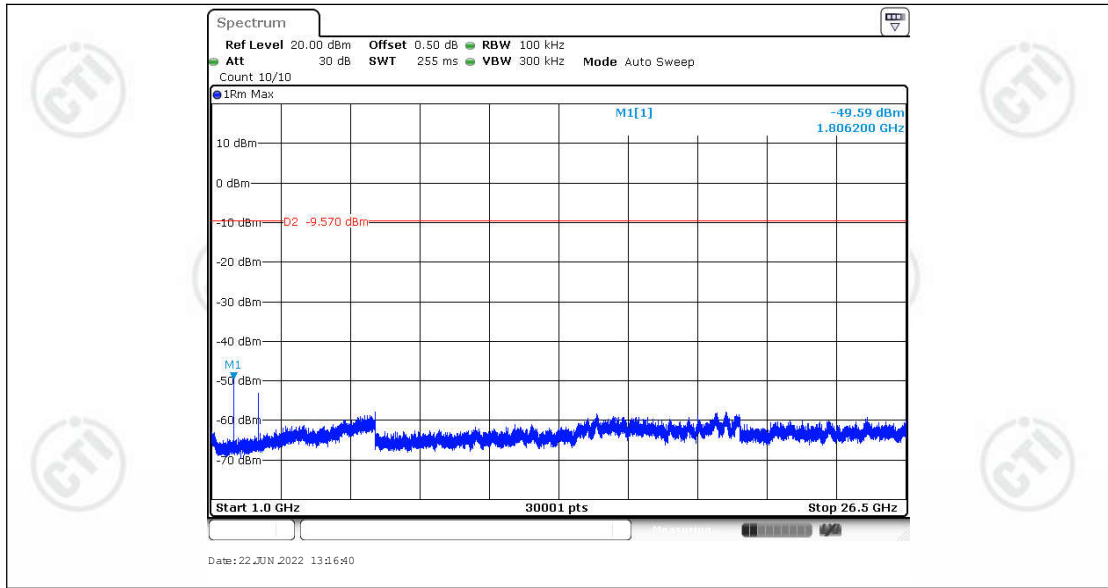
BW500K_Ant1_903_1000~26500
