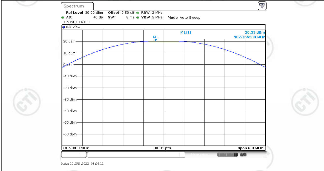
BW500K_Ant1_903
