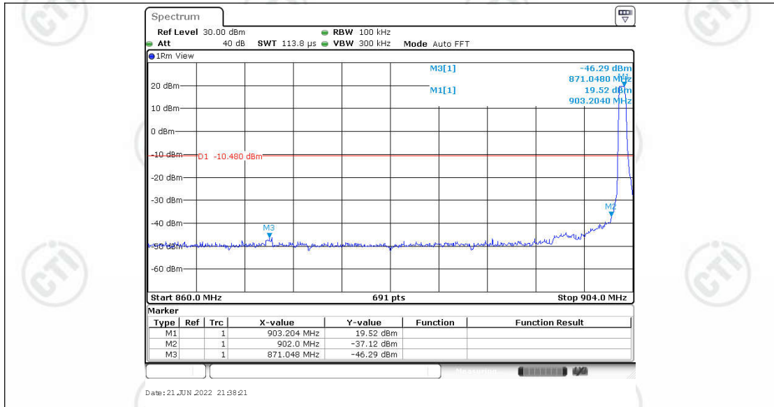
BW500K_Ant1_903
