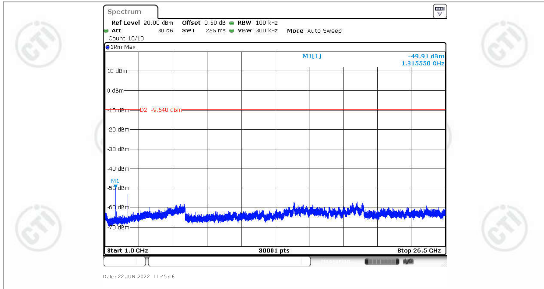
BW1523.4K_Ant1_907.8_1000~26500
