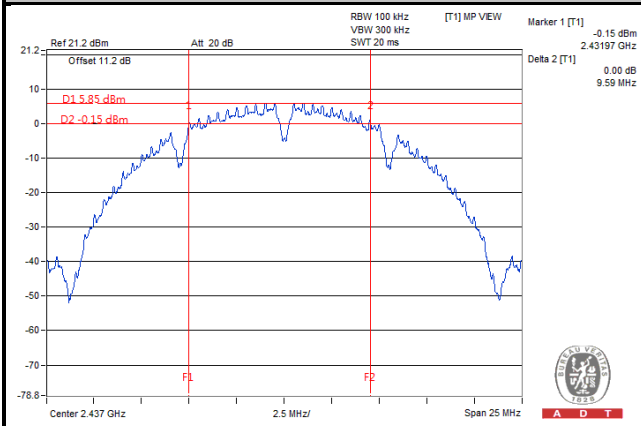
802.11n (20MHz)
