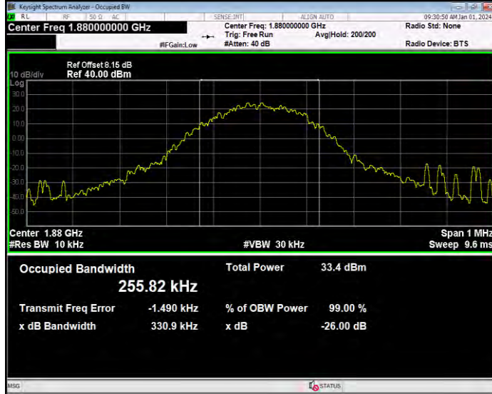
EGPRS1900 Channel=810
