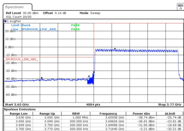
n77(3700-3980) SCS=30kHz DFT_QPSK BW=70MHz LowChannel=649000 RB=180@0
