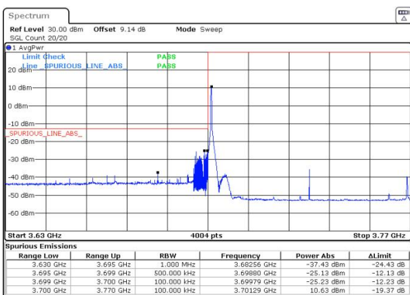
n77(3700-3980) SCS=30kHz DFT_QPSK BW=70MHz LowChannel=649000 RB=1@0
