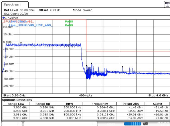
n77(3700-3980) SCS=30kHz DFT_16QAM BW=20MHz HighChannel=664666 RB=50@0
