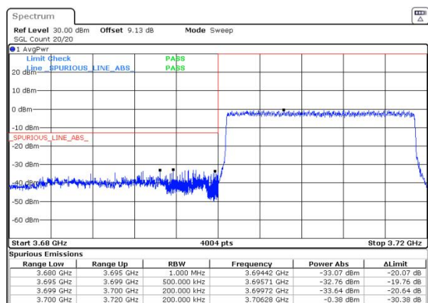
n77(3700-3980) SCS=30kHz DFT_BPSK BW=20MHz LowChannel=647334 RB=50@0
