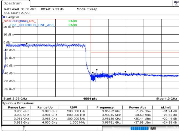
n77(3700-3980) SCS=30kHz DFT_16QAM BW=20MHz HighChannel=664666 RB=50@0
