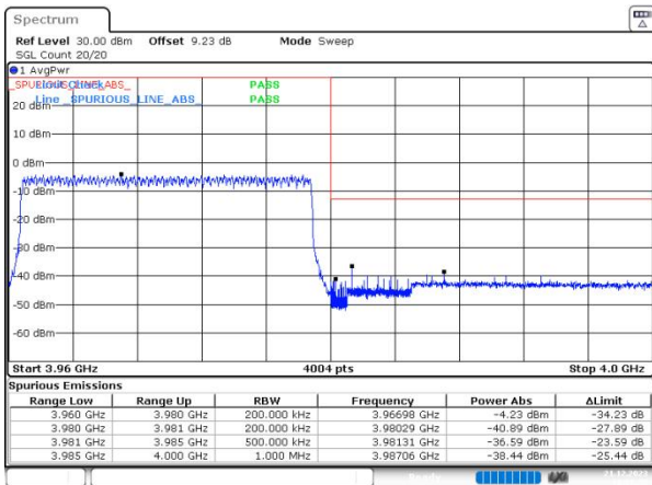
n77(3700-3980) SCS=30kHz DFT_64QAM BW=20MHz HighChannel=664666 RB=50@0
