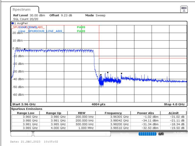
n77(3700-3980) SCS=30kHz DFT_QPSK BW=20MHz HighChannel=664666 RB=50@0
