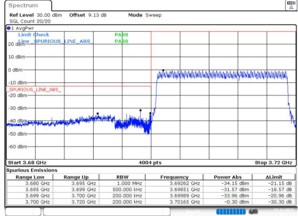
n77(3700-3980) SCS=30kHz DFT_16QAM BW=20MHz LowChannel=647334 RB=50@0
