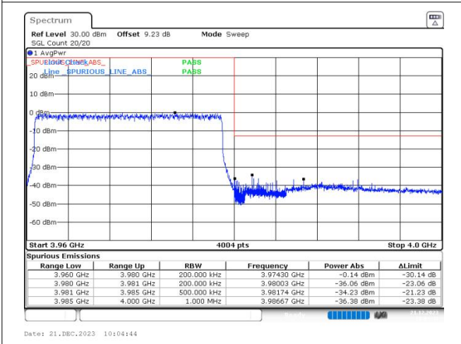
n77(3700-3980) SCS=30kHz DFT_BPSK BW=20MHz HighChannel=664666 RB=50@0
