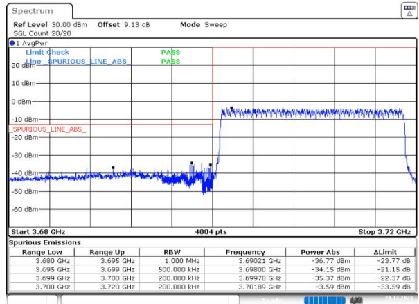
n77(3700-3980) SCS=30kHz DFT_64QAM BW=20MHz LowChannel=647334 RB=50@0
