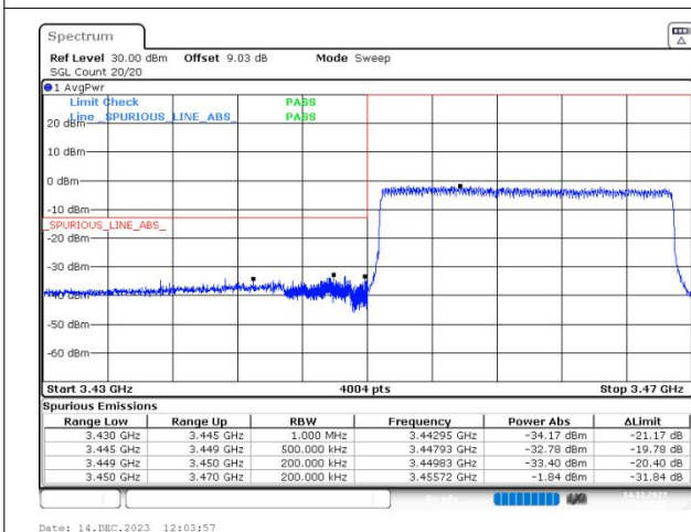
n78(3450-3550) SCS=30kHz DFT_QPSK BW=20MHz LowChannel=630668 RB=50@0
