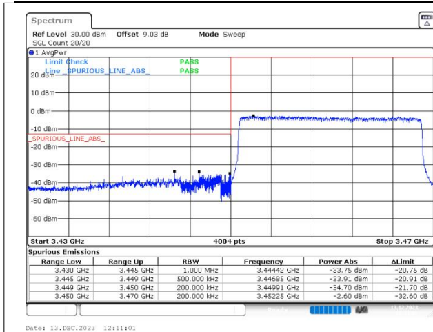
n77(3450-3550) SCS=30kHz DFT_16QAM BW=20MHz LowChannel=630668 RB=50@0
