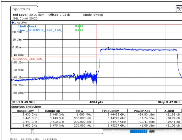
n77(3450-3550) SCS=30kHz DFT_QPSK BW=20MHz LowChannel=630668 RB=50@0
