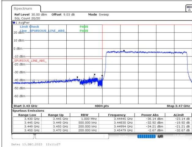
n77(3450-3550) SCS=30kHz DFT_64QAM BW=20MHz LowChannel=630668 RB=50@0
