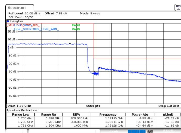
n66 SCS=15kHz DFT_QPSK BW=20MHz HighChannel=354000 RB=100@0
