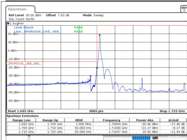
n66 SCS=15kHz DFT_16QAM BW=15MHz LowChannel=343500 RB=1@0
