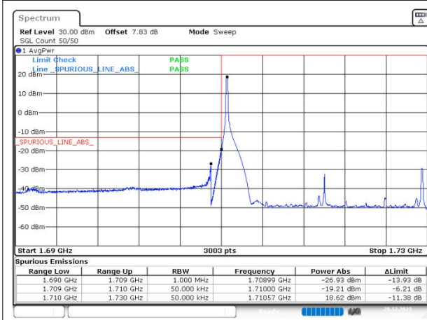
n66 SCS=15kHz DFT_QPSK BW=20MHz LowChannel=344000 RB=1@0
