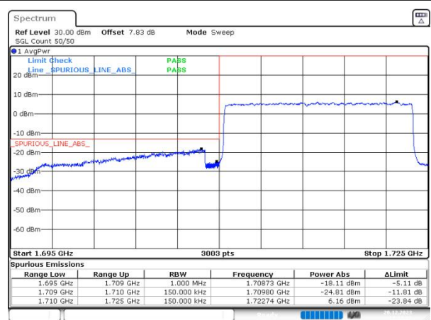
n66 SCS=15kHz DFT_BPSK BW=15MHz LowChannel=343500 RB=75@0
