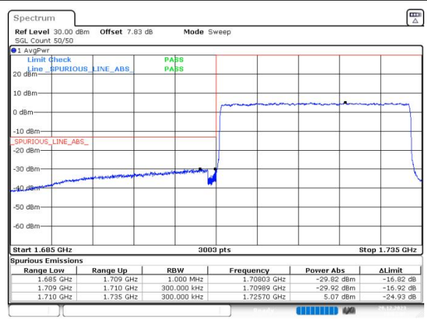
n66 SCS=15kHz DFT_16QAM BW=25MHz LowChannel=344500 RB=128@0
