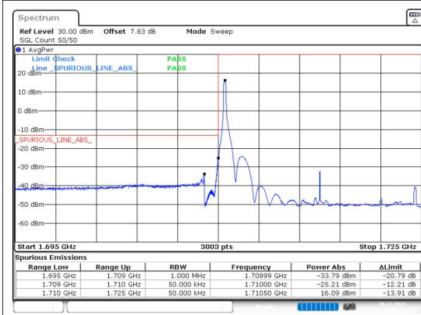
n66 SCS=15kHz DFT_64QAM BW=15MHz LowChannel=343500 RB=1@0
