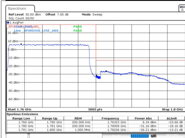
n66 SCS=15kHz DFT_BPSK BW=20MHz HighChannel=354000 RB=100@0
