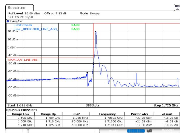
n66 SCS=15kHz DFT_BPSK BW=15MHz LowChannel=343500 RB=1@0
