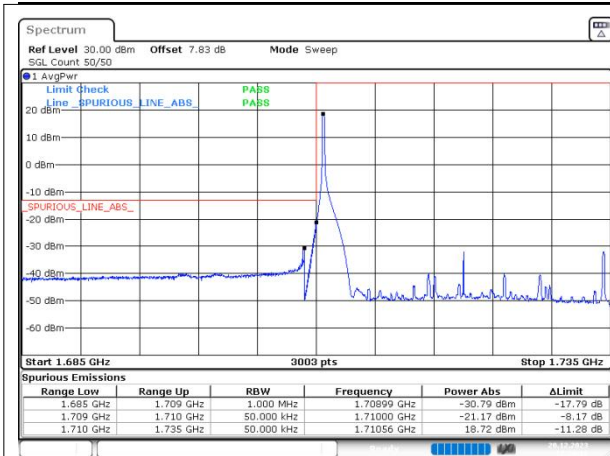
n66 SCS=15kHz DFT_QPSK BW=25MHz LowChannel=344500 RB=1@0
