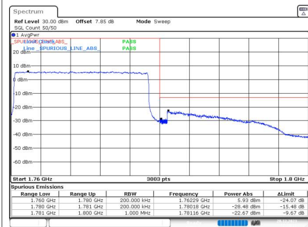
n66 SCS=15kHz DFT_BPSK BW=20MHz HighChannel=354000 RB=100@0
