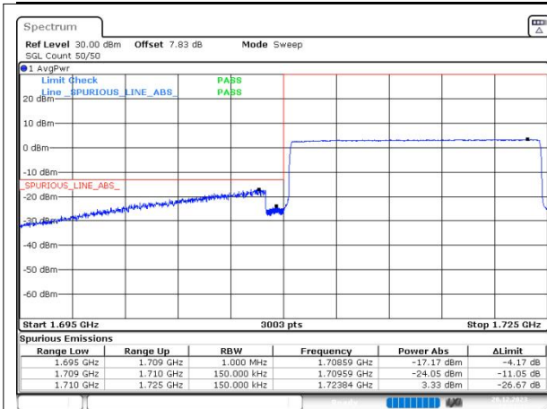
n66 SCS=15kHz CP_QPSK BW=15MHz LowChannel=343500 RB=79@0
