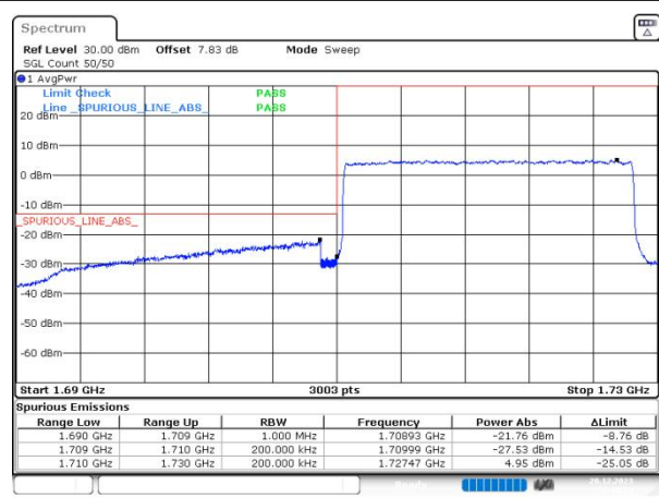
n66 SCS=15kHz DFT_QPSK BW=20MHz LowChannel=344000 RB=100@0
