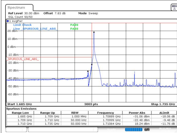
n66 SCS=15kHz DFT_16QAM BW=25MHz LowChannel=344500 RB=1@0
