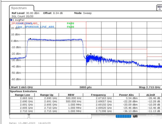
n41 SCS=30kHz DFT_QPSK BW=20MHz HighChannel=535998 RB=50@0
