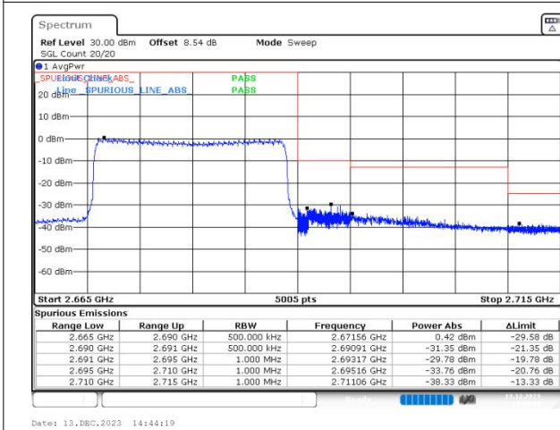
n41 SCS=30kHz DFT_256QAM BW=20MHz HighChannel=535998 RB=50@0
