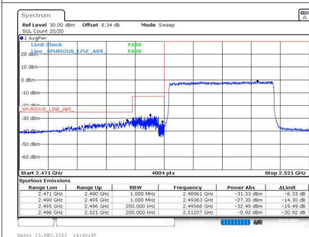
n41 SCS=30kHz DFT_QPSK BW=20MHz LowChannel=501204 RB=50@0
