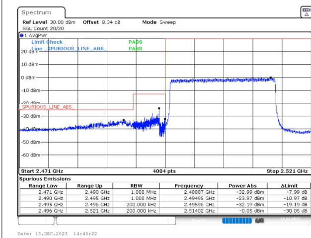
n41 SCS=30kHz DFT_BPSK BW=20MHz LowChannel=501204 RB=50@0
