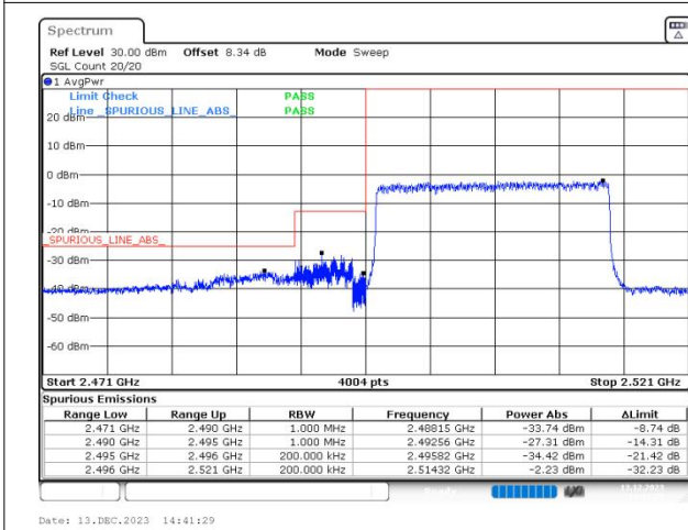
n41 SCS=30kHz DFT_64QAM BW=20MHz LowChannel=501204 RB=50@0
