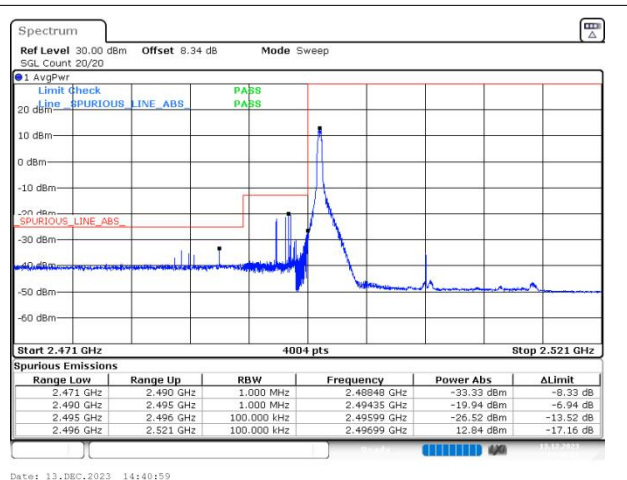
n41 SCS=30kHz DFT_QPSK BW=20MHz LowChannel=501204 RB=1@0
