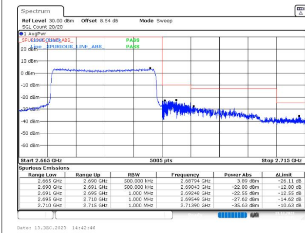
n41 SCS=30kHz DFT_BPSK BW=20MHz HighChannel=535998 RB=50@0
