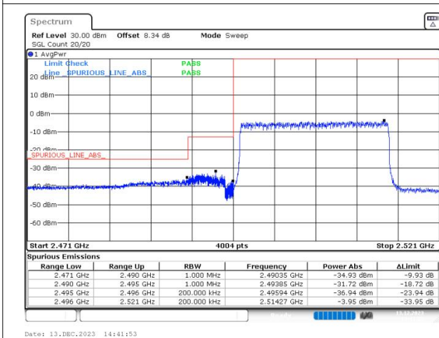
n41 SCS=30kHz DFT_256QAM BW=20MHz LowChannel=501204 RB=50@0
