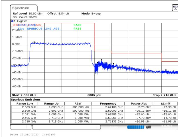
n41 SCS=30kHz DFT_64QAM BW=20MHz HighChannel=535998 RB=50@0
