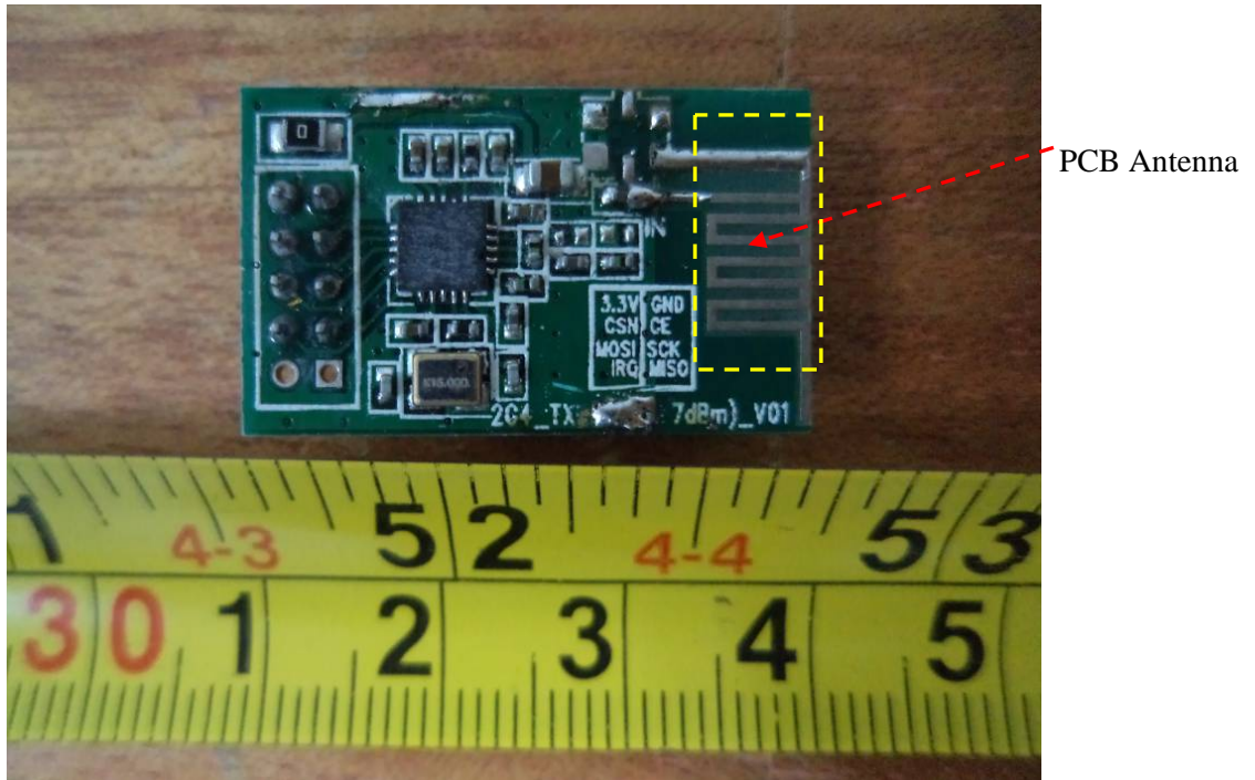
EUT –RF Module Bottom View
