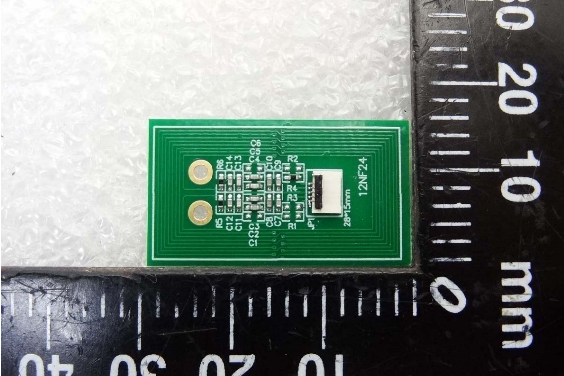
EUT 14 Antenna
