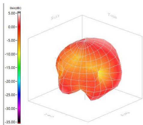
5.85GHz
