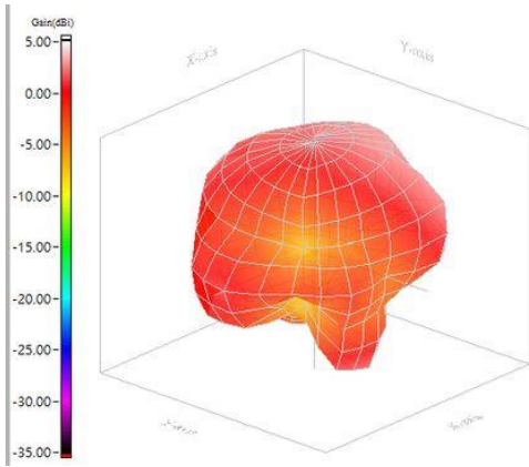
5.35GHz
