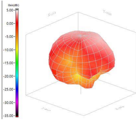
5.15GHz
