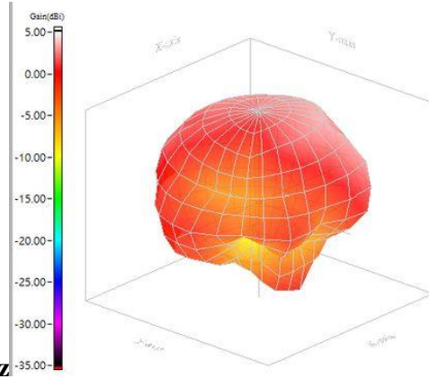
5.25GHz
