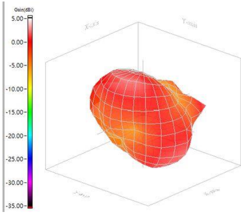
2.5GHz
