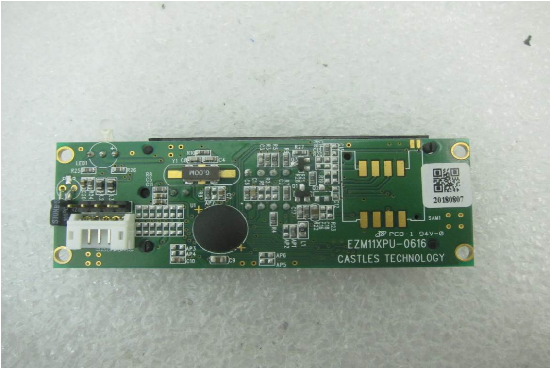
EUT 69 27P-RM-2
