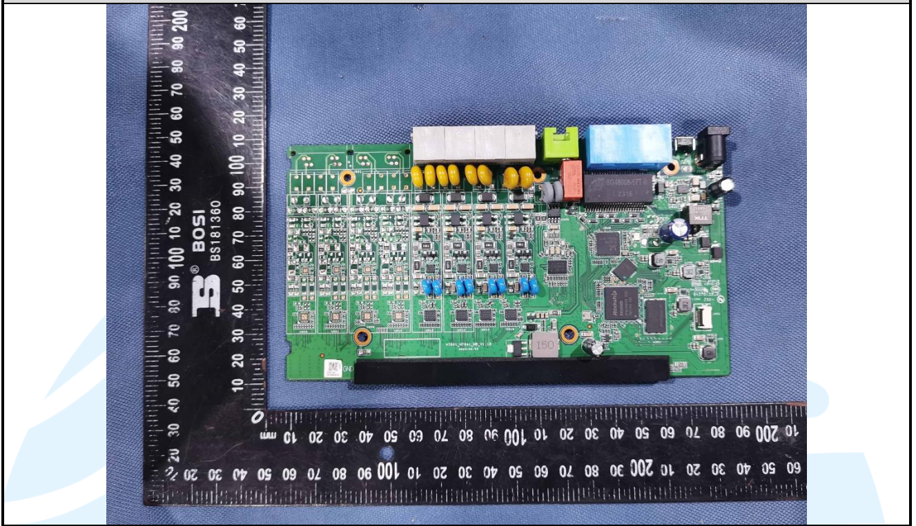
EUT Photo(HT841)
