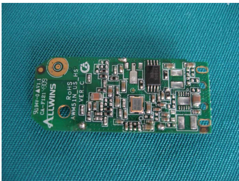
802.11b/g/n module -Rear View
