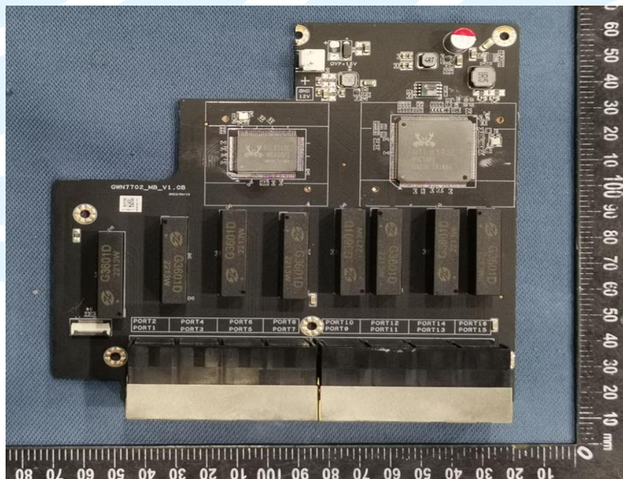
EUT Photo
