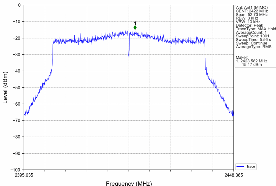
802.11be(EHT40)_LCH_2422MHz_SU_Ant1 (MIMO)_NTNV
