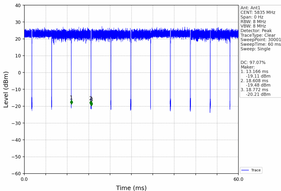
802.11n(HT40)_HCH_5835MHz_Ant1_NTNV
