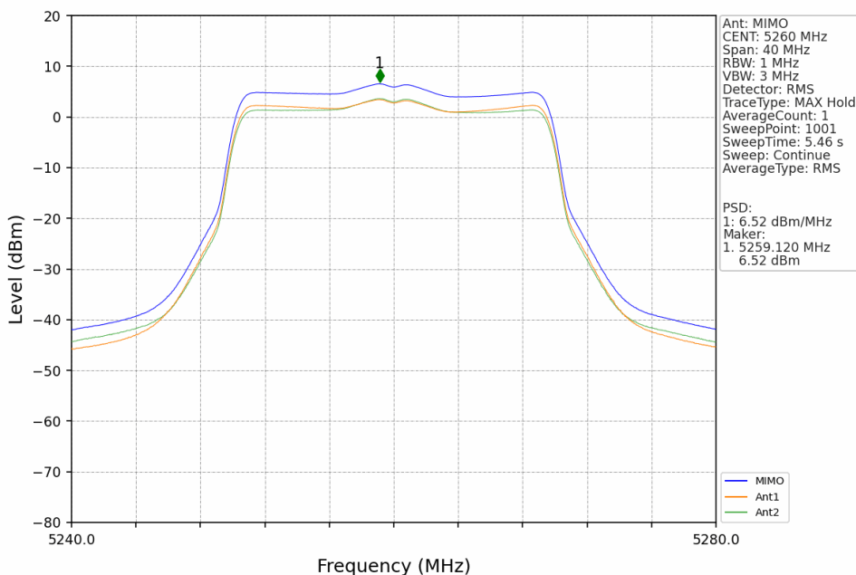
802.11be(EHT20)_LCH_5260MHz_SU_MIMO_NTNV
