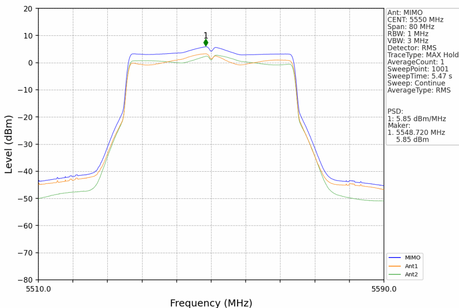
802.11be(EHT40)_MCH_5550MHz_SU_MIMO_NTNV
