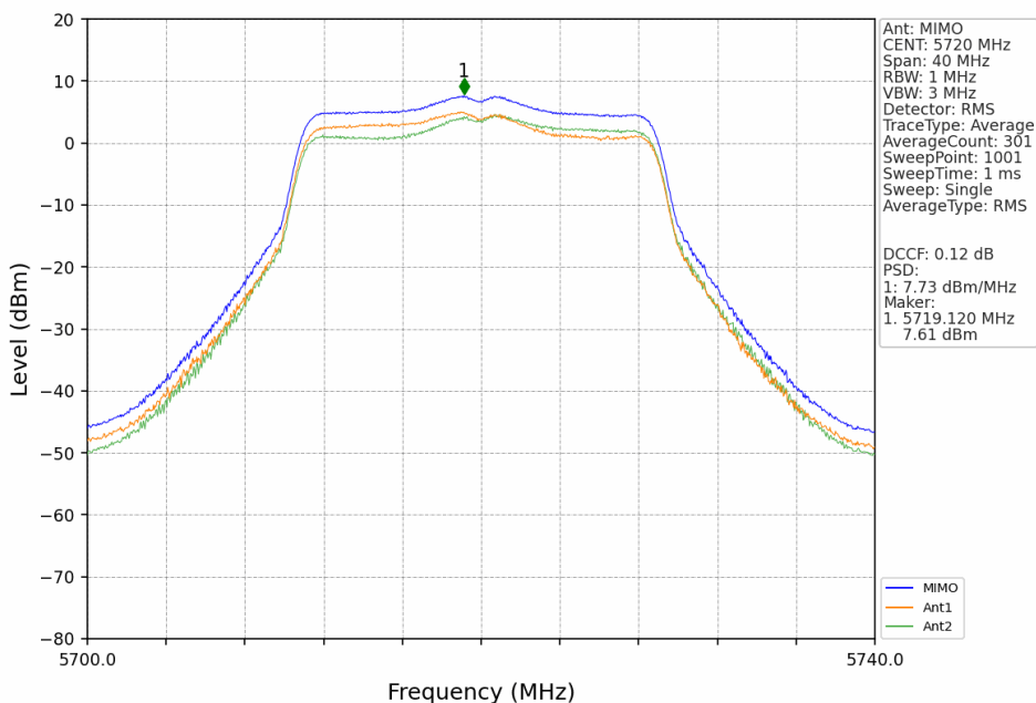
802.11n(HT20)_HCH_5720MHz_MIMO_NTNV
