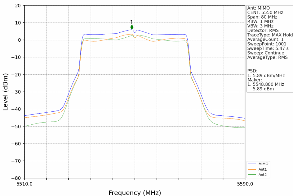
802.11ax(HEW40)_MCH_5550MHz_SU_MIMO_NTNV
