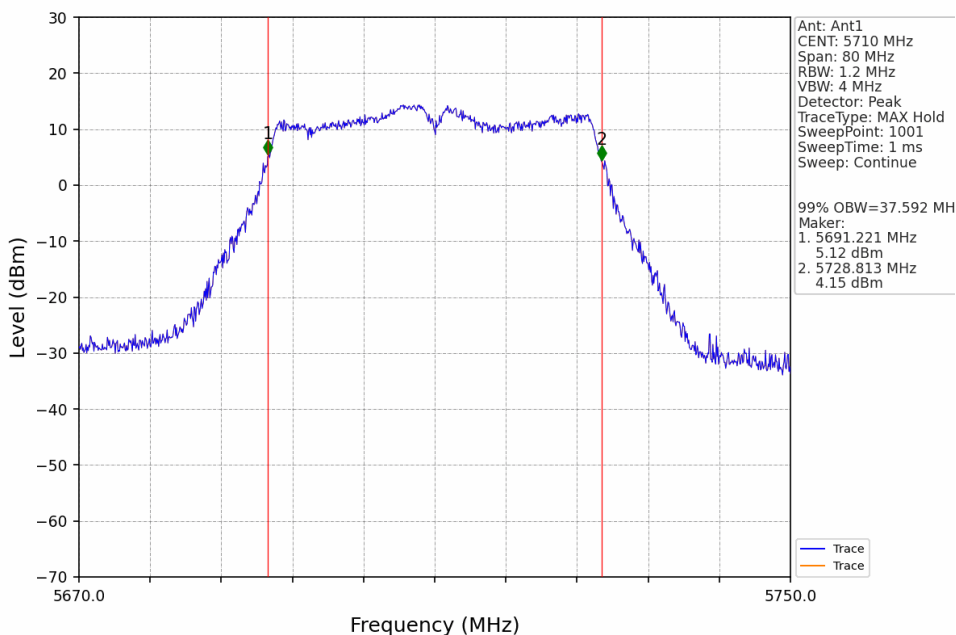
802.11n(HT40)_HCH_5710MHz_Ant1_NTNV
