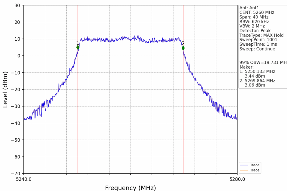
802.11be(EHT20)_LCH_5260MHz_SU_Ant1_NTNV
