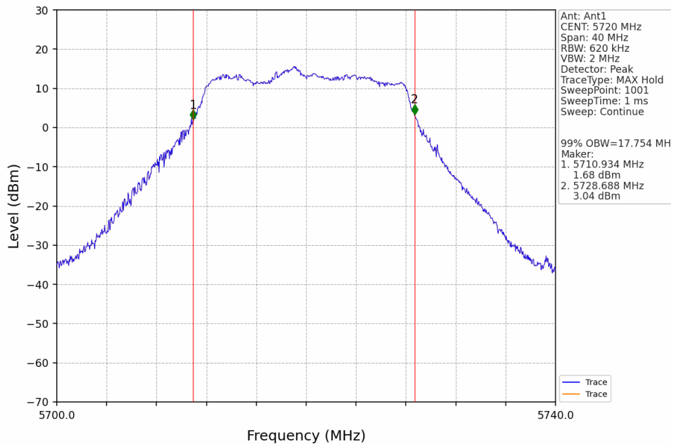
802.11a_HCH_5720MHz_Ant1_NTNV
