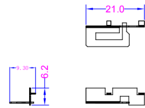
6G Antenna
