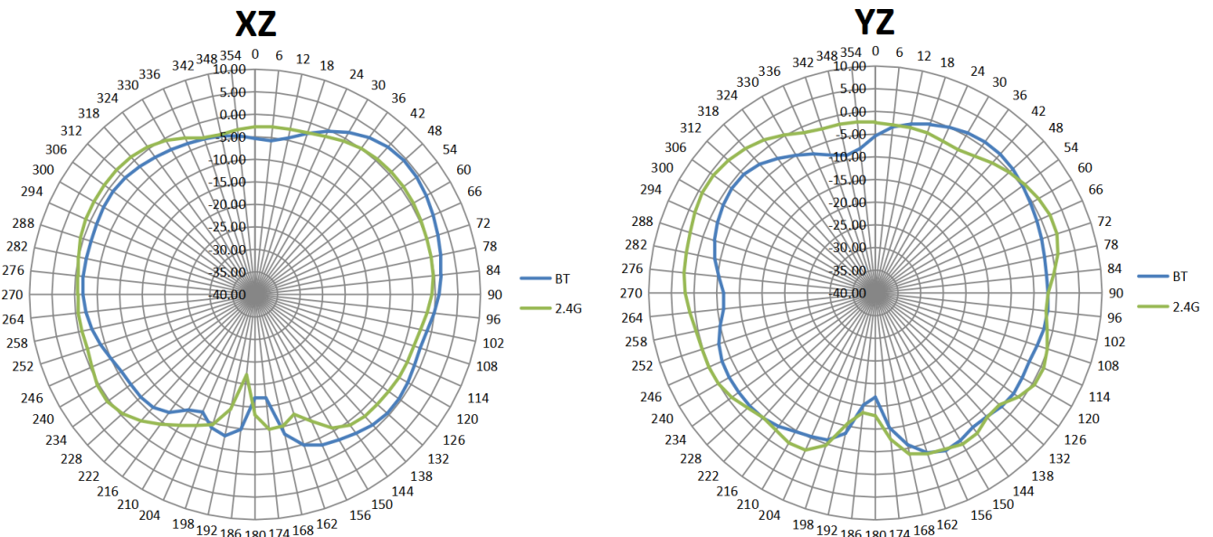
BT/2.4G 辐射方向图 Radiation Patterns(unit:dB)
