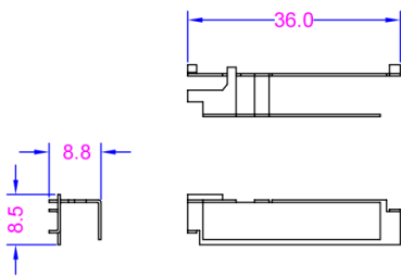
2.4G Antenna
