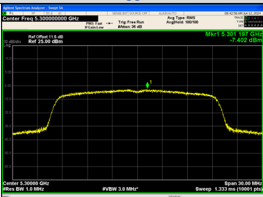
IEEE 802.11ax_Channel 60_20MHz_Antenna 2_RU&Index SU
