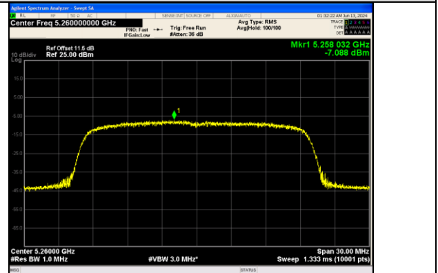
IEEE 802.11ax_Channel 52_20MHz_Antenna 3_RU&Index SU
