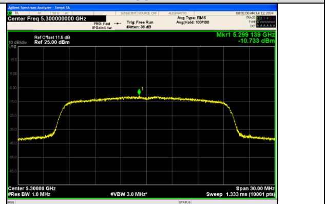
IEEE 802.11ax_Channel 60_20MHz_Antenna 1_RU&Index SU
