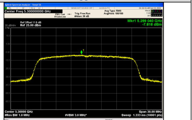
IEEE 802.11ax_Channel 60_20MHz_Antenna 3_RU&Index SU
