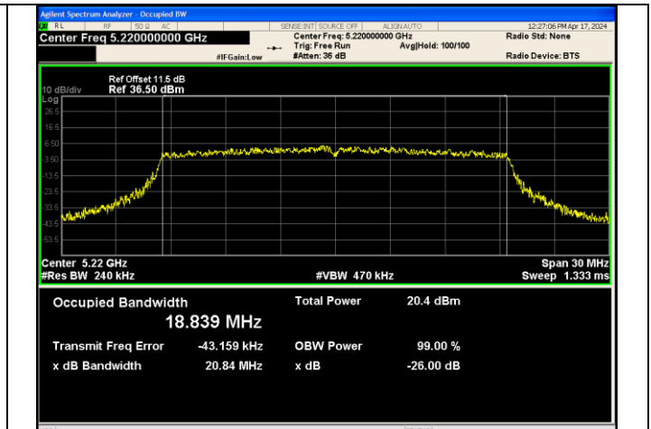
IEEE 802.11ax_Channel 44_20MHz_Antenna 3_RU&Index SU
