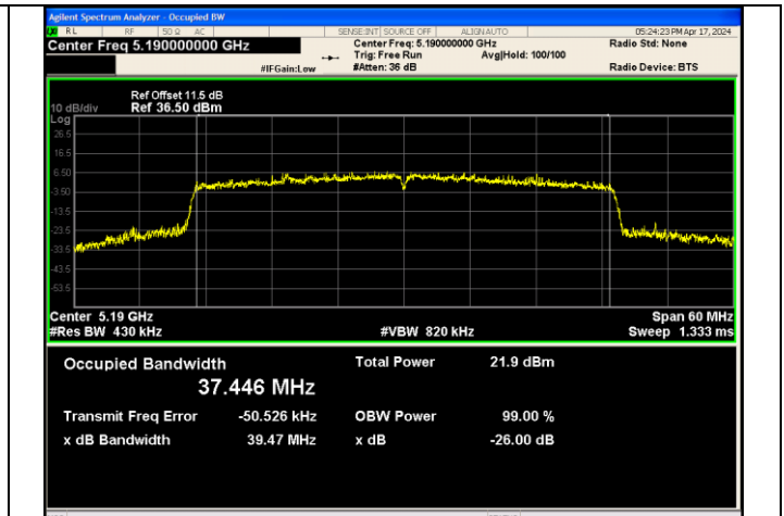
IEEE 802.11ax_Channel 38_40MHz_Antenna 1_RU&Index SU
