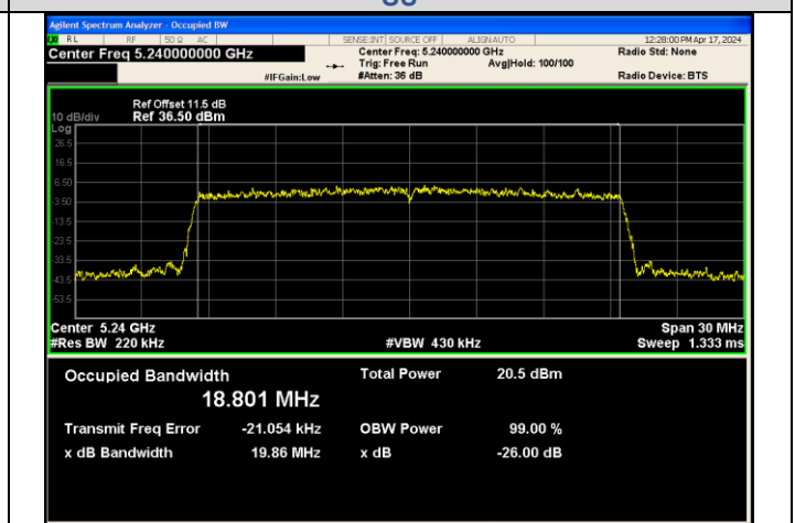
IEEE 802.11ax_Channel 48_20MHz_Antenna 3_RU&Index SU
