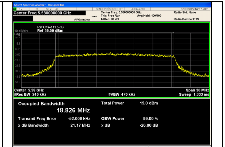
IEEE 802.11ax_Channel 116_20MHz_Antenna 3_RU&Index SU
