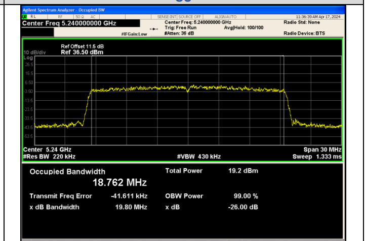
IEEE 802.11ax_Channel 48_20MHz_Antenna 1_RU&Index SU
