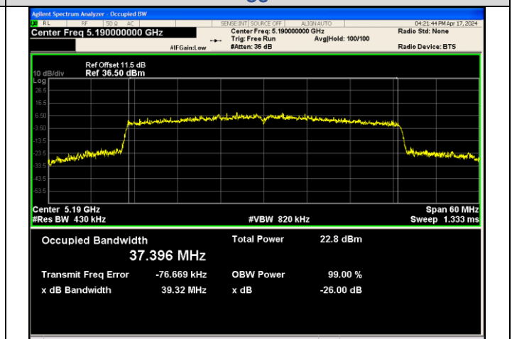
IEEE 802.11ax_Channel 38_40MHz_Antenna 3_RU&Index SU
