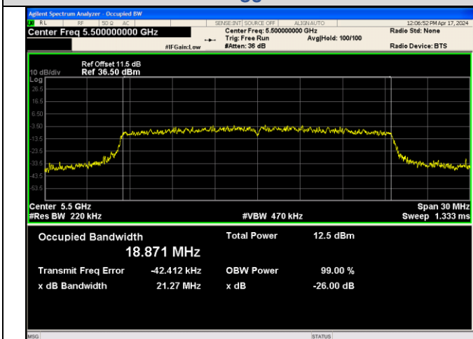
IEEE 802.11ax_Channel 100_20MHz_Antenna 2_RU&Index SU
