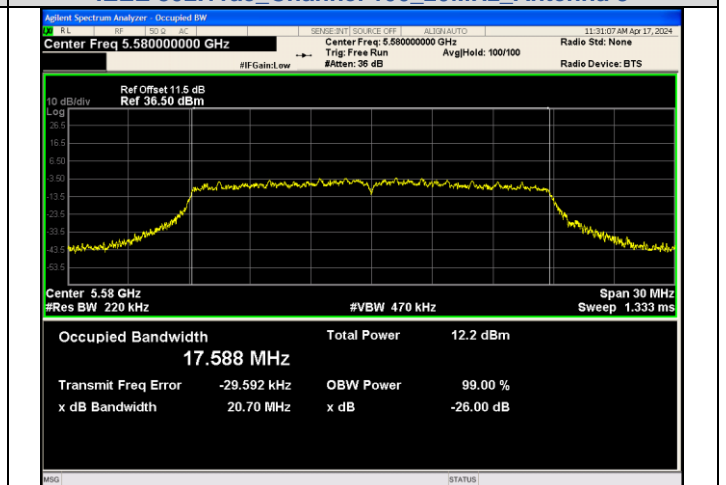
IEEE 802.11ac_Channel 116_20MHz_Antenna 1
