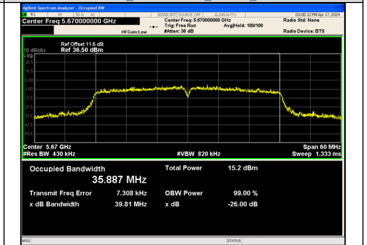
IEEE 802.11n_Channel 134_40MHz_Antenna 3
