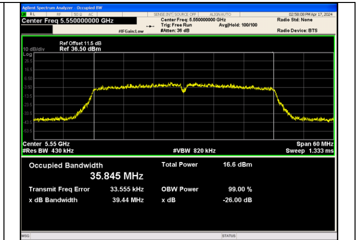
IEEE 802.11n_Channel 110_40MHz_Antenna 3
