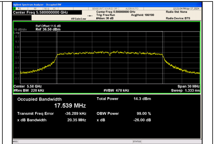
IEEE 802.11ac_Channel 116_20MHz_Antenna 3
