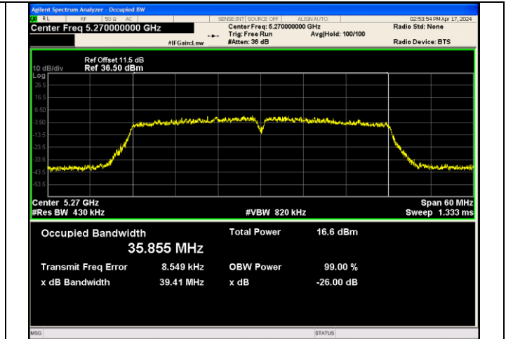
IEEE 802.11n_Channel 54_40MHz_Antenna 3
