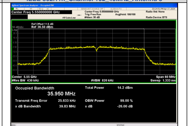
IEEE 802.11n_Channel 110_40MHz_Antenna 1
