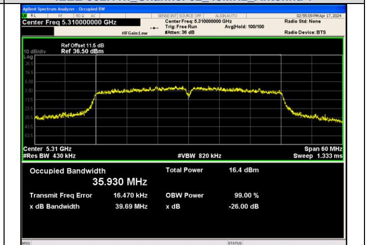
IEEE 802.11n_Channel 62_40MHz_Antenna 3
