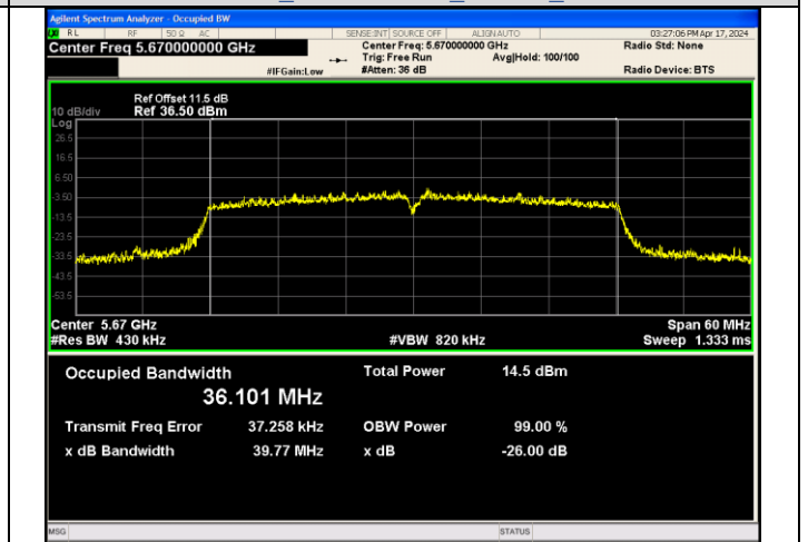
IEEE 802.11n_Channel 134_40MHz_Antenna 1
