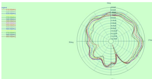
theta=90deg
