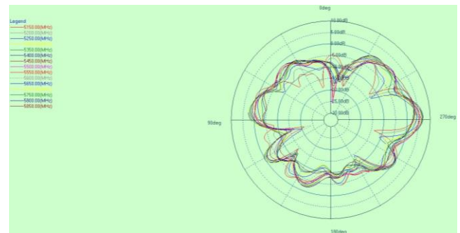
phi=90deg
