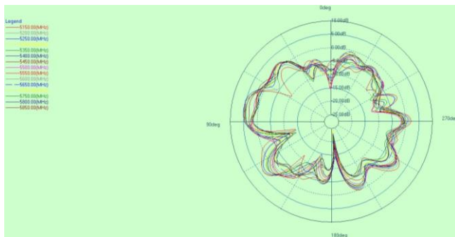
phi=0deg
