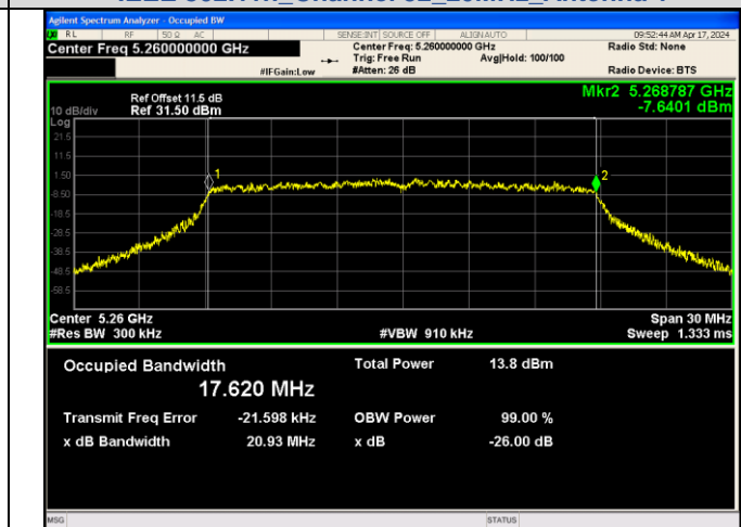
IEEE 802.11n_Channel 52_20MHz_Antenna 3
