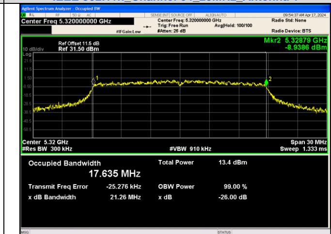
IEEE 802.11n_Channel 64_20MHz_Antenna 3
