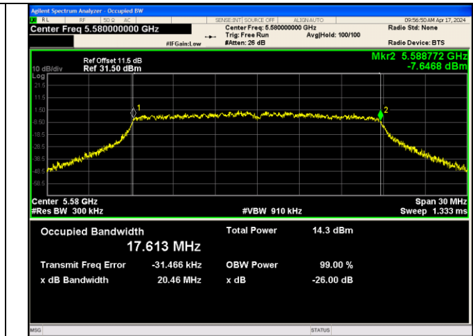
IEEE 802.11n_Channel 116_20MHz_Antenna 3
