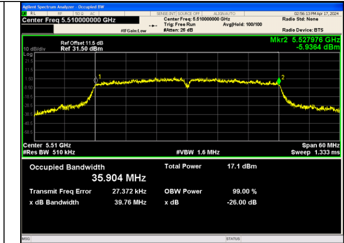
IEEE 802.11n_Channel 102_40MHz_Antenna 3
