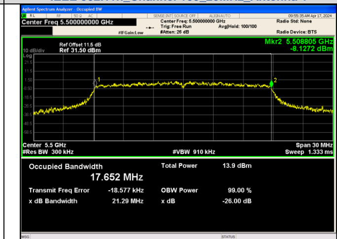
IEEE 802.11n_Channel 100_20MHz_Antenna 3
