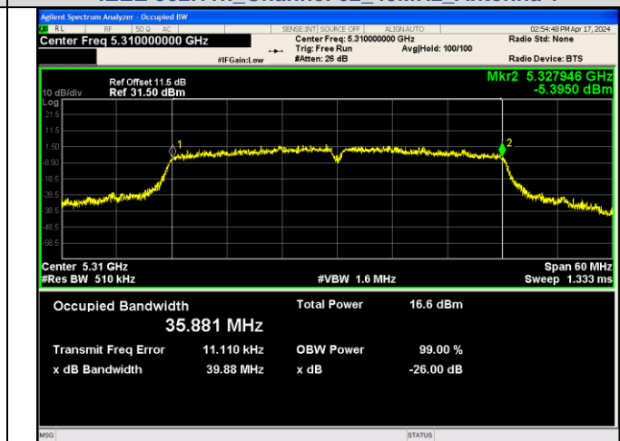
IEEE 802.11n_Channel 62_40MHz_Antenna 3
