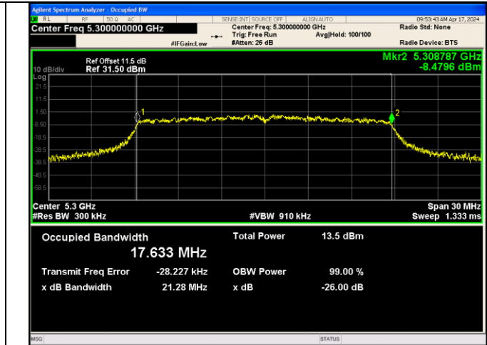
IEEE 802.11n_Channel 60_20MHz_Antenna 3
