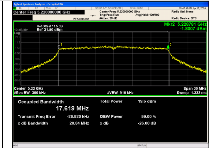
IEEE 802.11n_Channel 44_20MHz_Antenna 3
