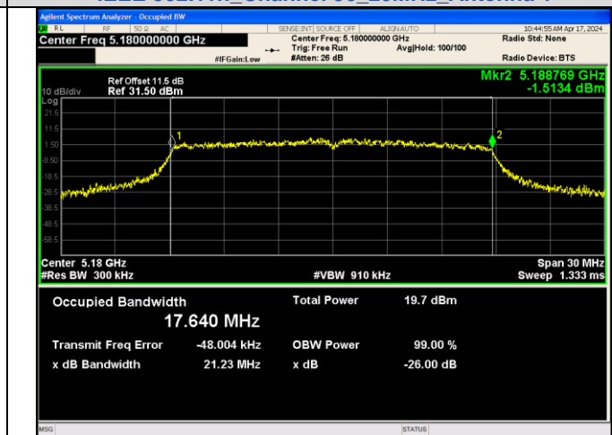
IEEE 802.11n_Channel 36_20MHz_Antenna 3
