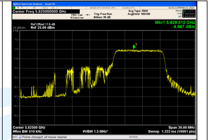
IEEE 802.11ax_Channel 165_20MHz_Antenna 3_RU&Index 52RU40
