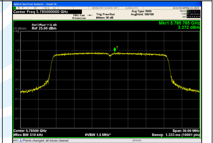
IEEE 802.11ax_Channel 157_20MHz_Antenna 1_RU&Index SU
