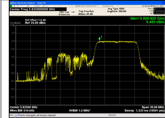
IEEE 802.11ax_Channel 165_20MHz_Antenna 0_RU&Index 52RU40
