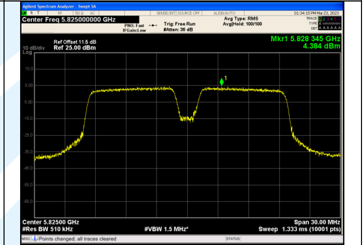
IEEE 802.11ax_Channel 165_20MHz_Antenna 1_RU&Index 106RU54
