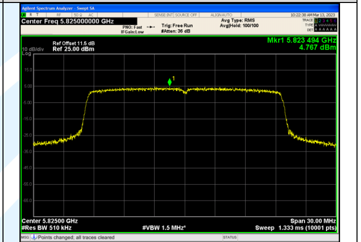
IEEE 802.11ax_Channel 165_20MHz_Antenna 1_RU&Index SU
