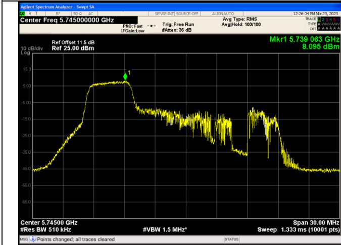
IEEE 802.11ax_Channel 149_20MHz_Antenna 0_RU&Index 26RU
