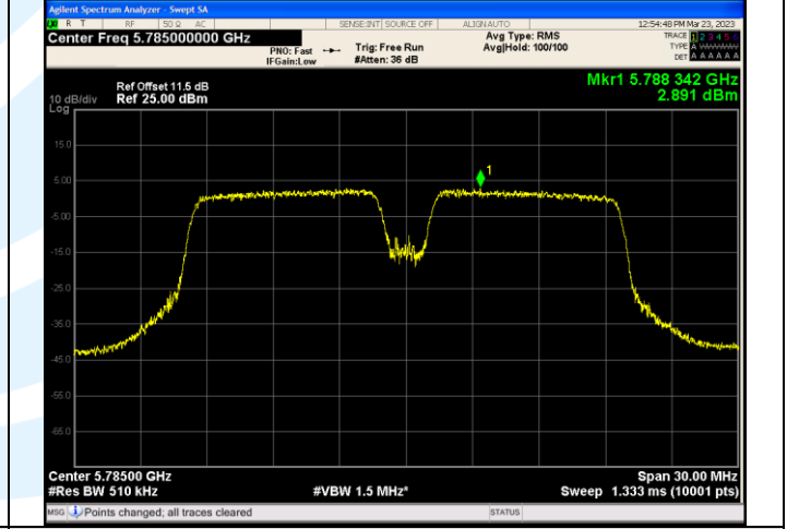
IEEE 802.11ax_Channel 157_20MHz_Antenna 1_RU&Index 106RU53
