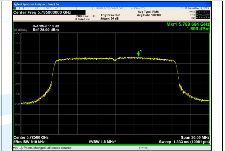
IEEE 802.11ax_Channel 157_20MHz_Antenna 3_RU&Index SU
